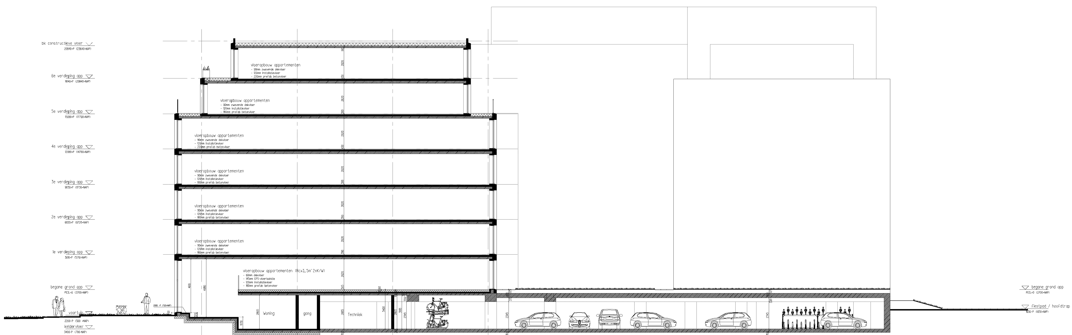
DOORSNEDE C-C
