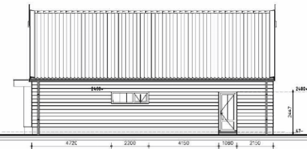
achtergevel
