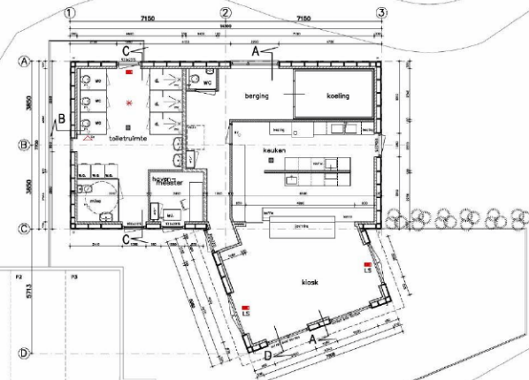
begane grond
