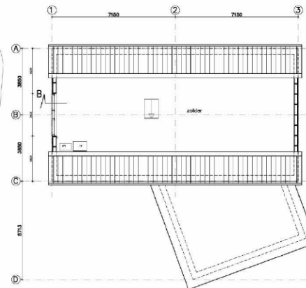
verdieping
