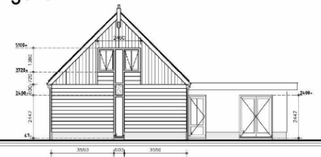
linker zijgevel
