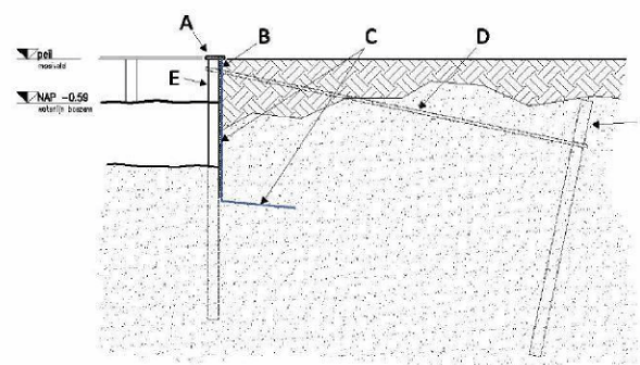
Doorsnede A - A
