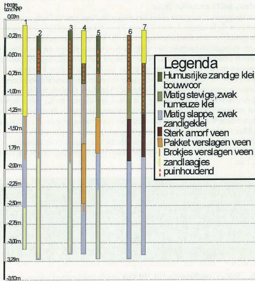
Figuur 6. Kolhorn, Westfriesedijk 154. Boorprofielen.
