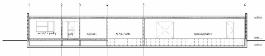
doorsnede A-A 1/100
