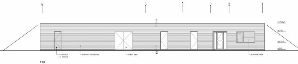
OOSTGEVEL 1/100
