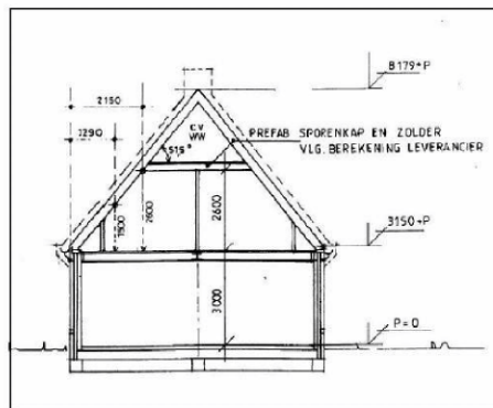
afb. 15 Doorsnede
