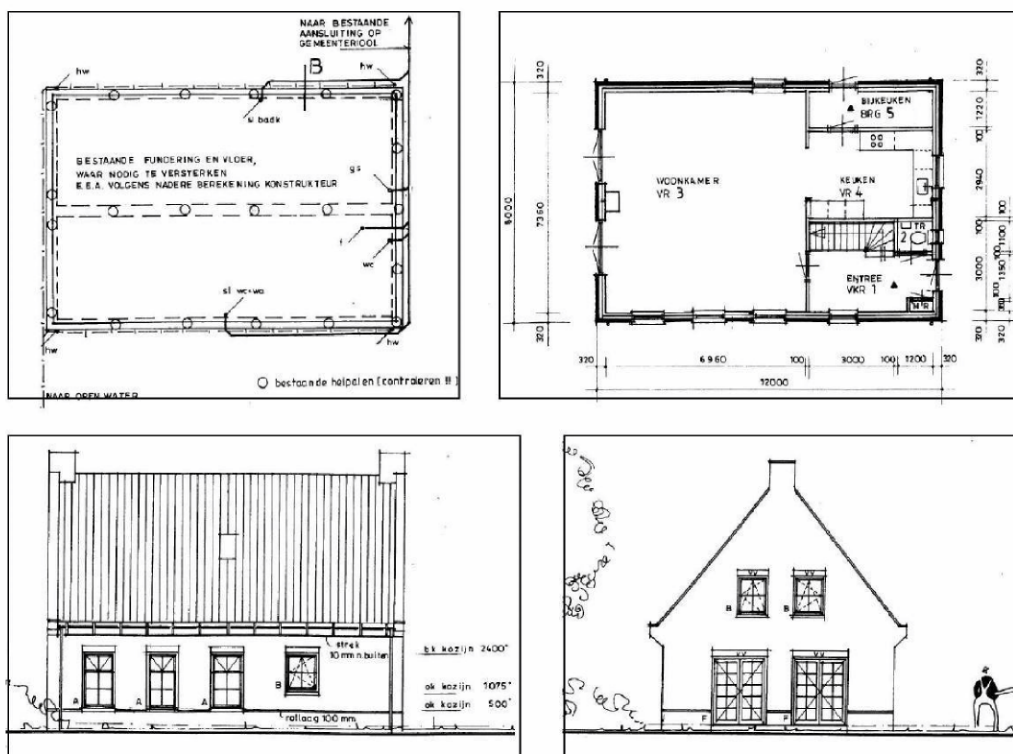
afb. 10, 11, 12 en 13 Fundering (bestaand), beganegrond en aanzichten dienstwoning.
