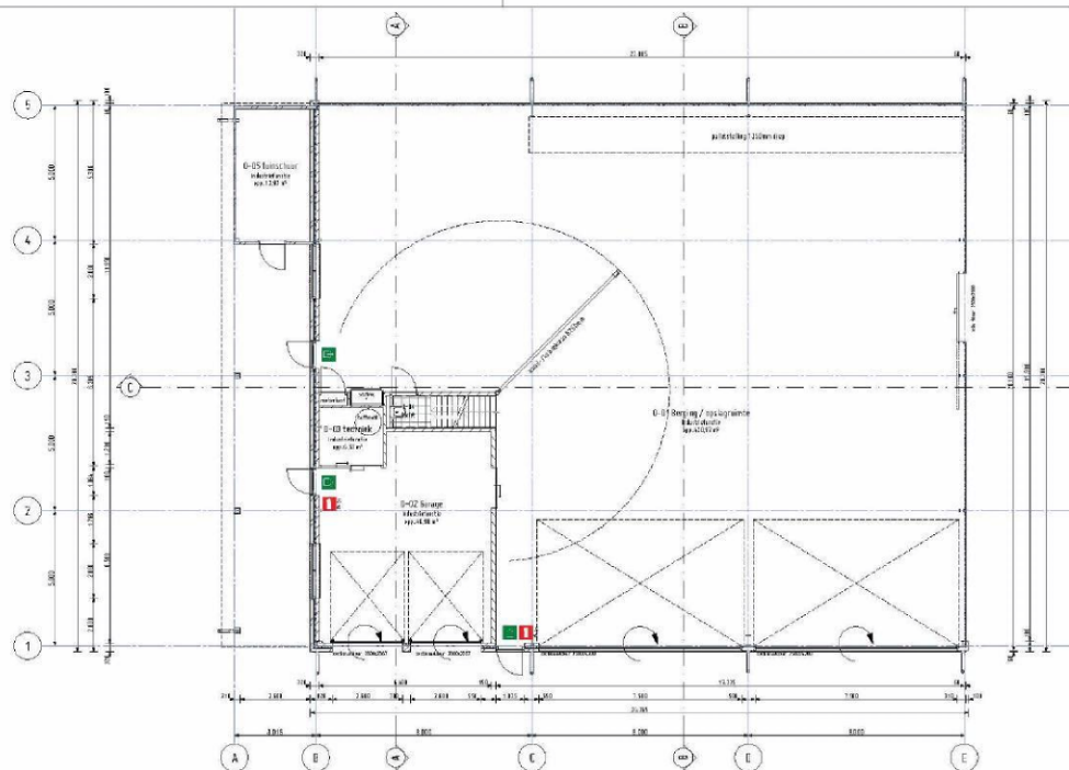
Begane grond 1:100
