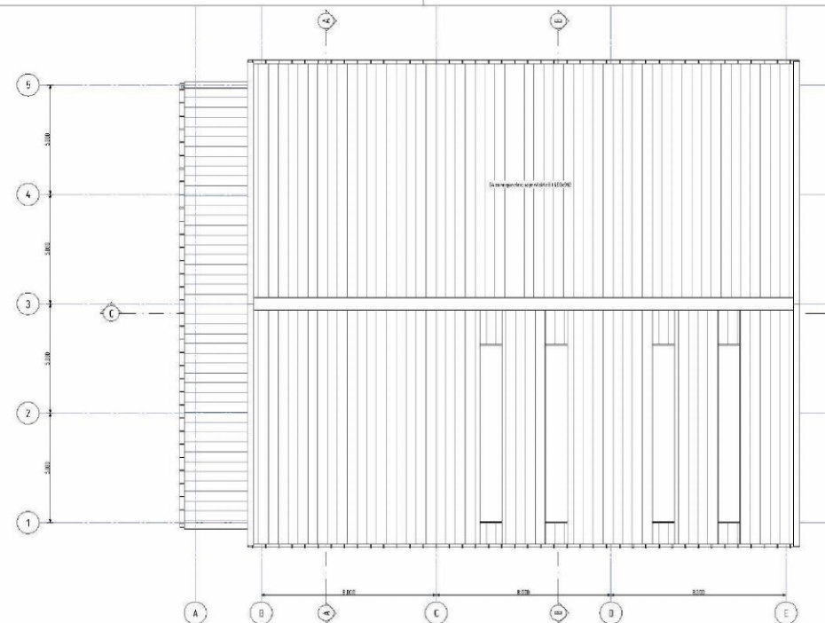
Dakoverzicht 1:100
