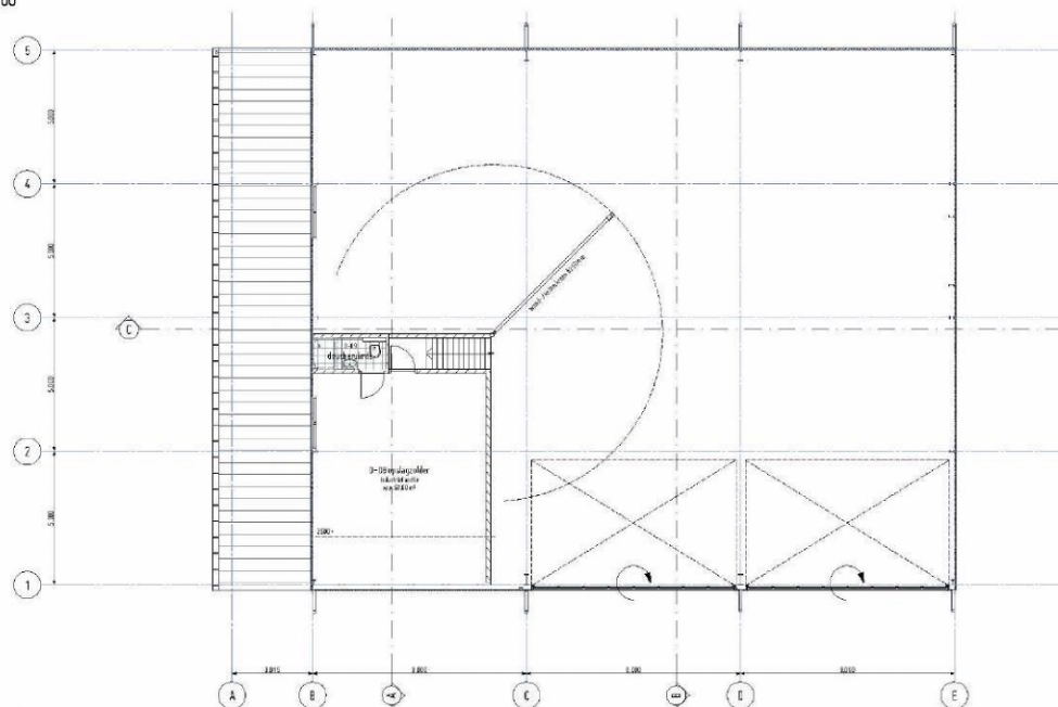
1e verdieping 1:100
