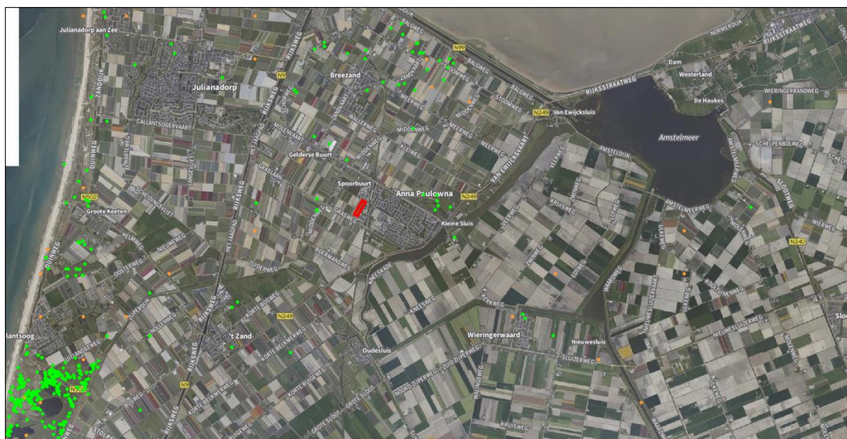
Figuur 2.9. Uit de omgeving van het plangebied (rood omlijnd), waaronder uit een sloot op minder dan een kilometer afstand van het plangebied zijn waarnemingen van rugstreepkikker (stippen) bekend (bron: NDFF).
