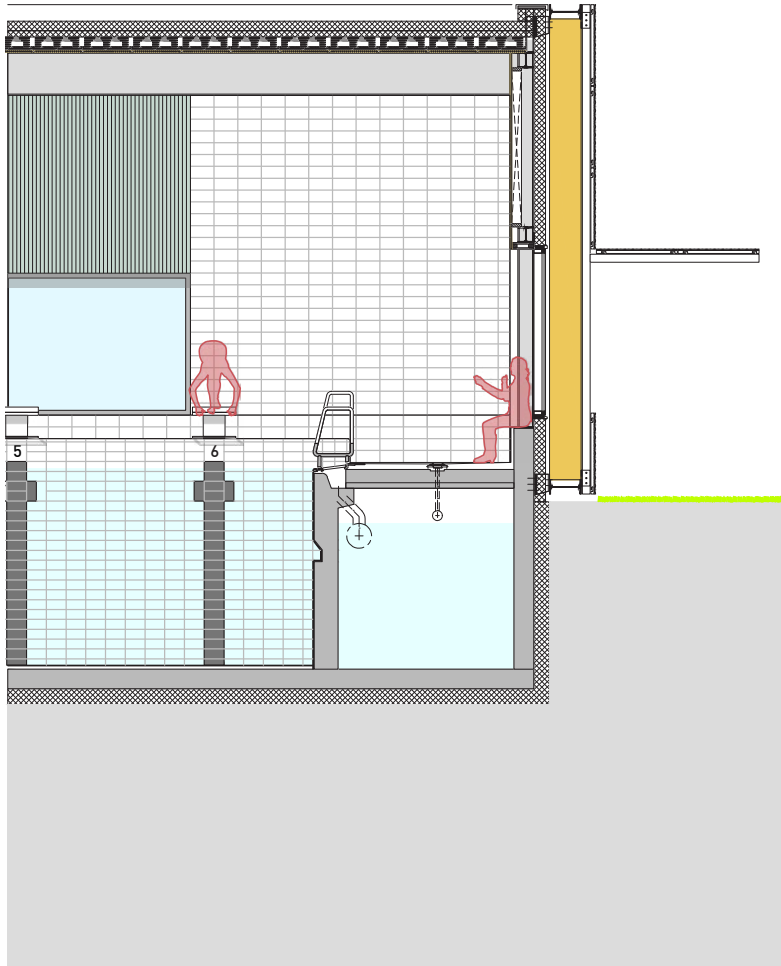
1: doorsnede.
