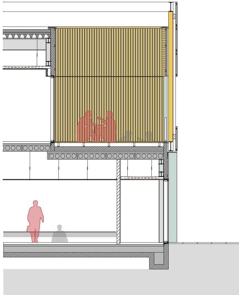
1: doorsnede.
