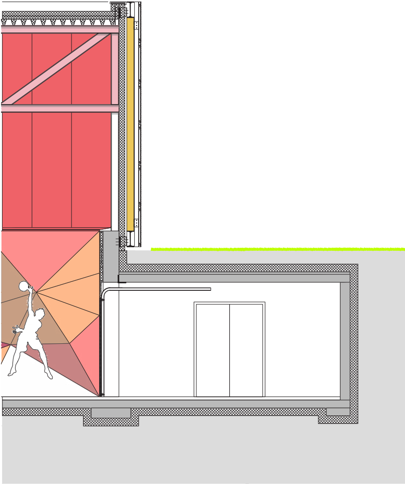
1: doorsnede.
