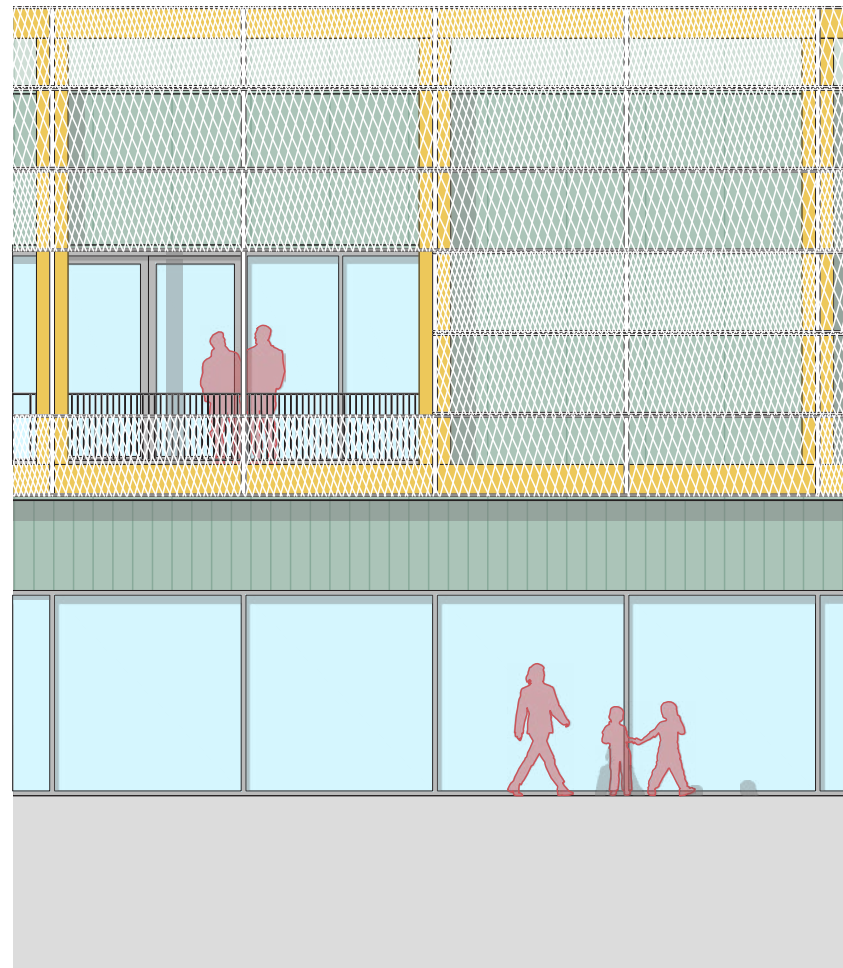
2: aanzicht.
