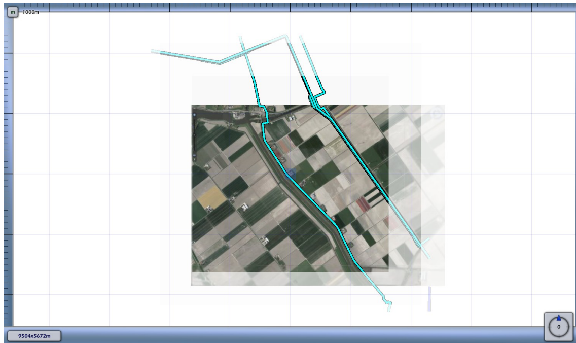
3.6 Figuur 3.6 Plaatsgebonden risico voor 4740_leiding-A-616-deel-2 van N.V. Nederlandse Gasunie
