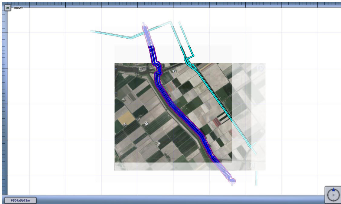
3.8 Figuur 3.8 Plaatsgebonden risico voor 4740_leiding-W-574-14-deel-1 van N.V. Nederlandse Gasunie
