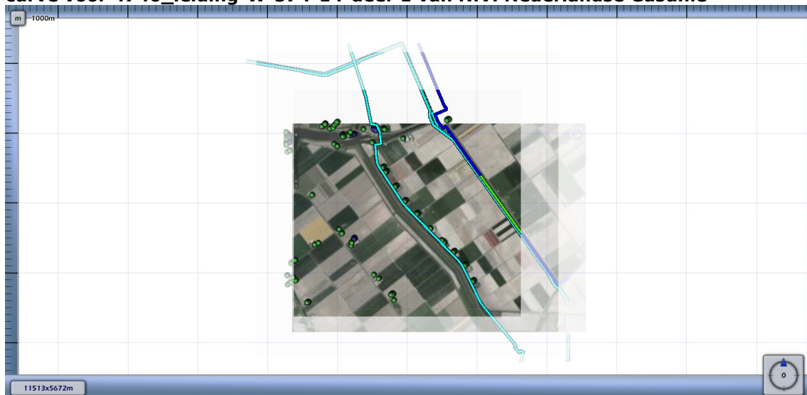
Figuur 4.8 Kilometer leiding behorende bij de maximale overschrijding van de FN-curve voor 4740_leiding-W-574-14-deel-1 van N.V. Nederlandse Gasunie
