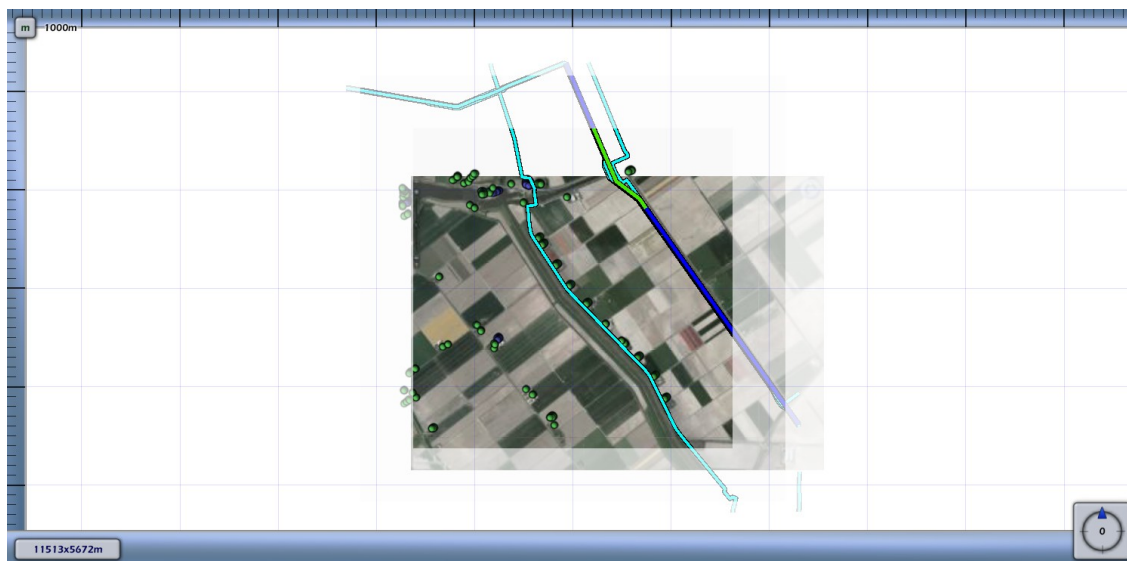
4.4 Figuur 4.4 Groepsrisico screening voor 4740_leiding-A-593-deel-2 van N.V. Nederlandse Gasunie
