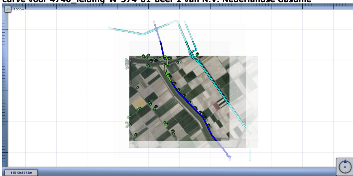
Figuur 4.7 Kilometer leiding behorende bij de maximale overschrijding van de FN-curve voor 4740_leiding-W-574-01-deel-1 van N.V. Nederlandse Gasunie
