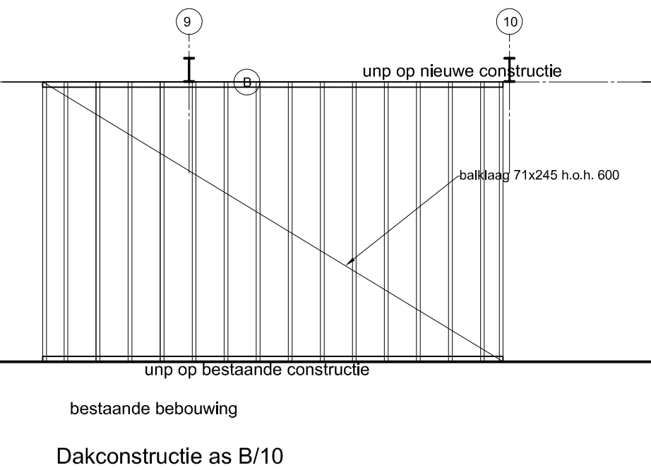
Dakconstructie as B/10
