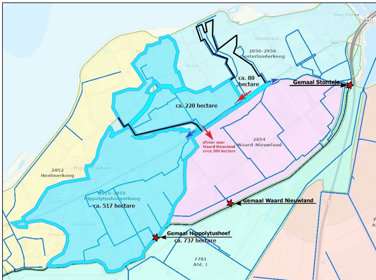
Afbeelding 12: Schematische weergave bemalingsgebied gemaal Hippolytushoef
