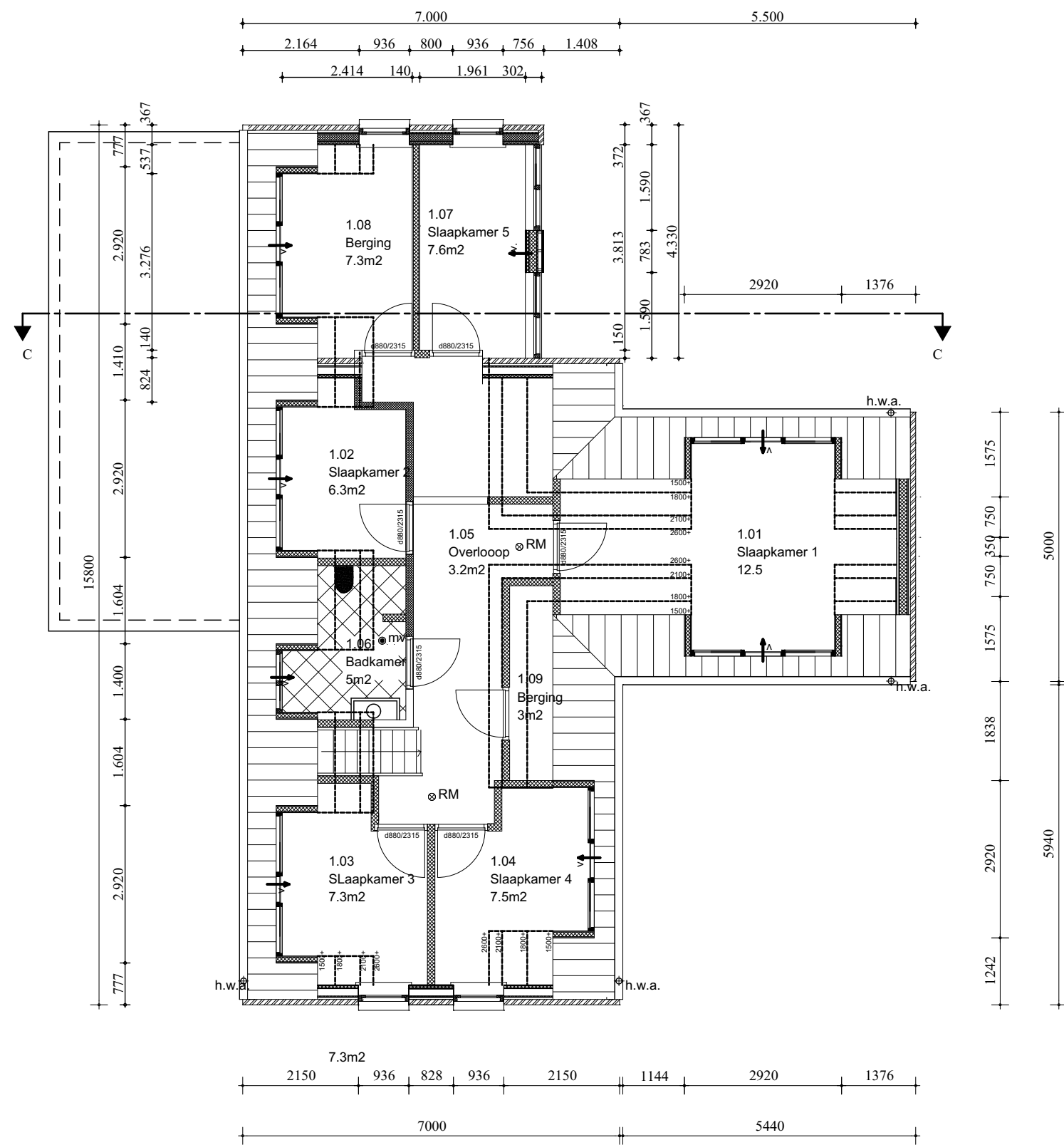
Plattegrond 1e verdieping
