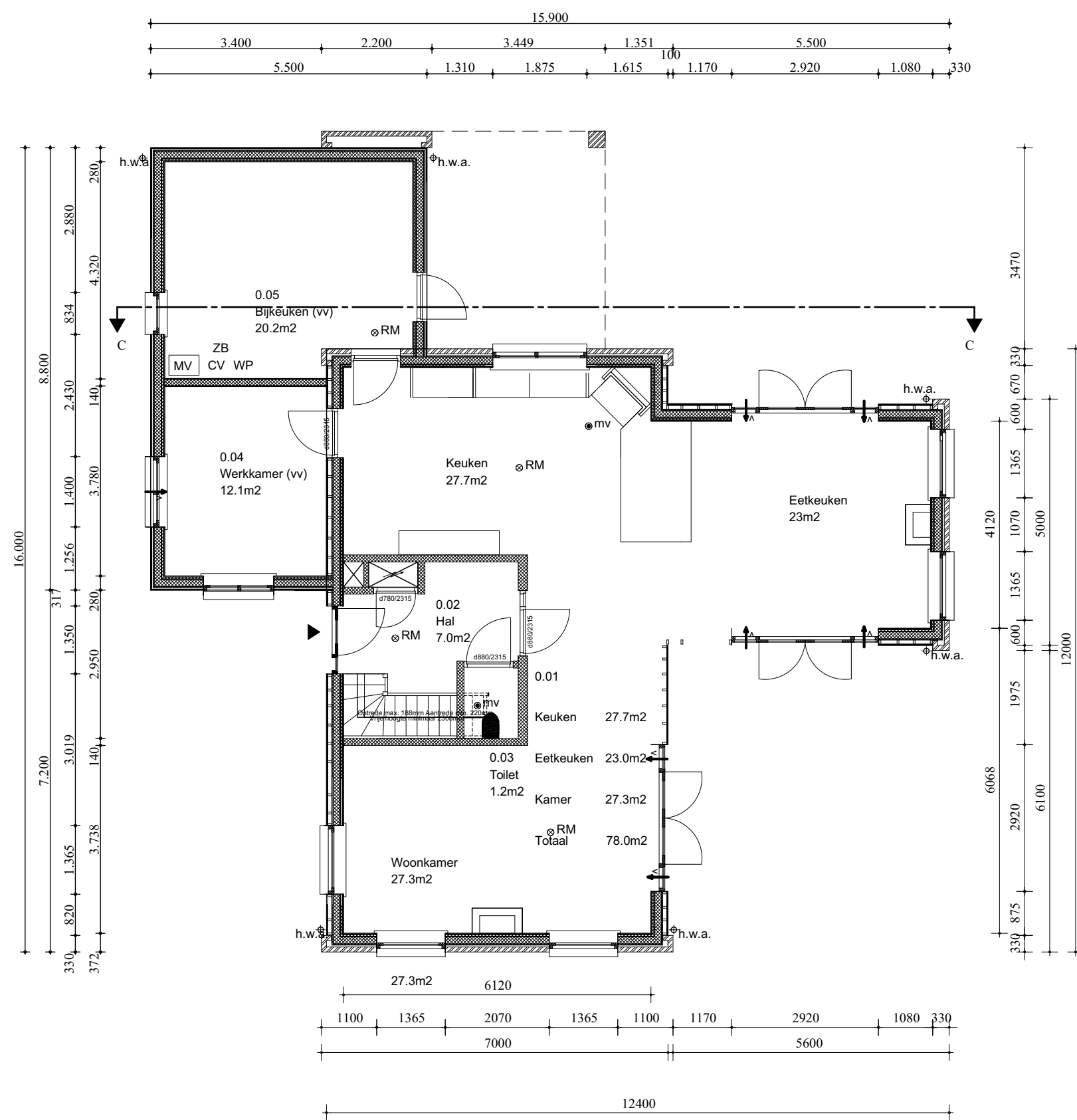
Plattegrond Begane Grond
