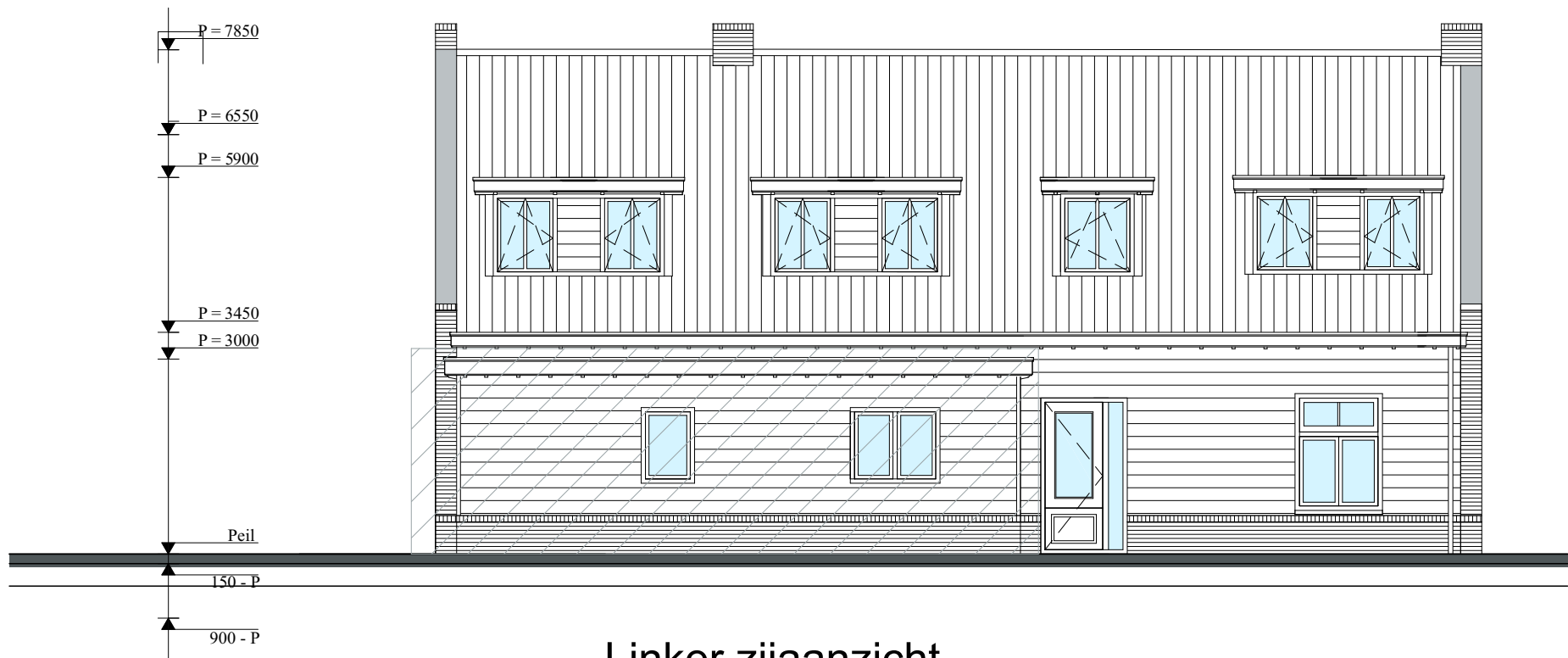
Linker zijaanzicht
