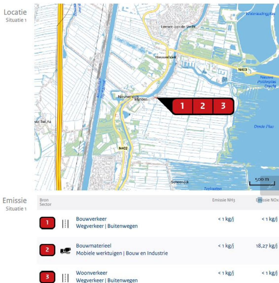
Figuur 3. Aeriusberekening met invoer verkeersbewegingen en gebruik mobiele werktuigen
