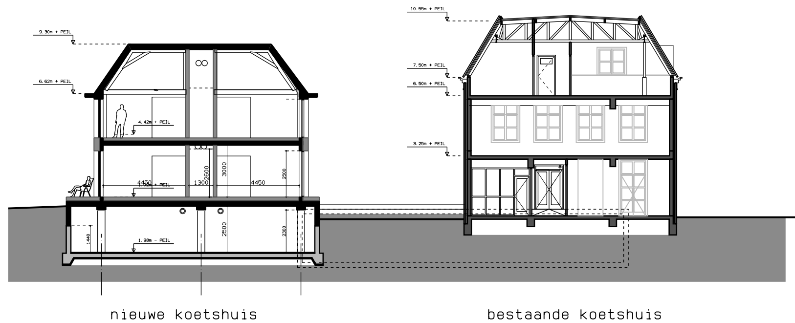
Dwarsdoorsnede
