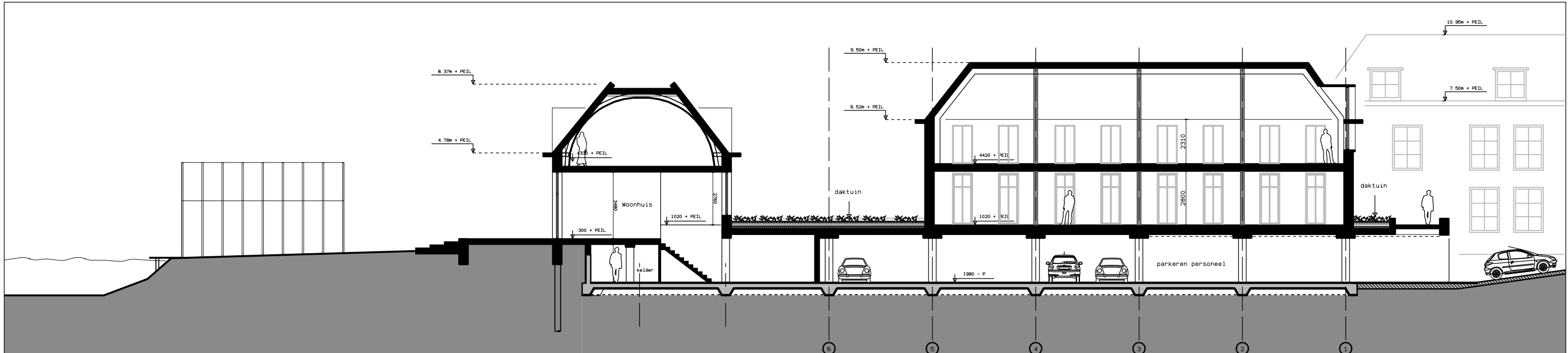
Langsdoorsnede
