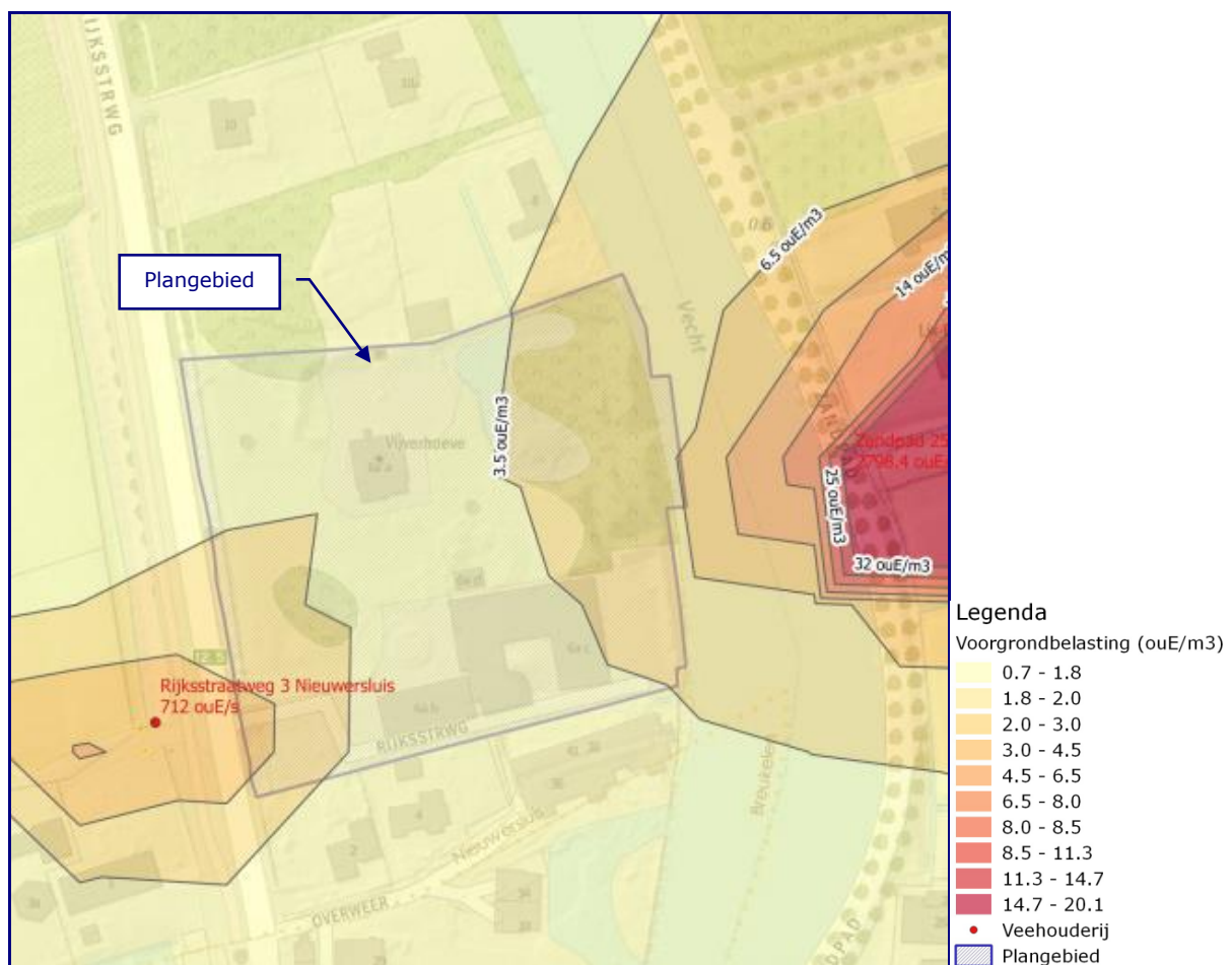
Afbeelding 9. Geurcontouren achtergrondbelasting
