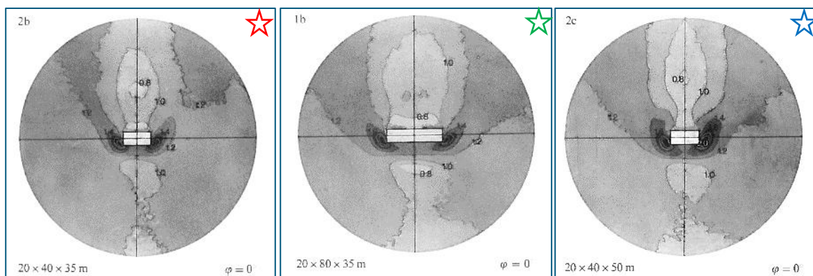
Afbeelding 5-2 Strooming rond een 40m breed en 35m hoog gebouw. De windrichting in de afbeeldingen is van onder naar boven 2
