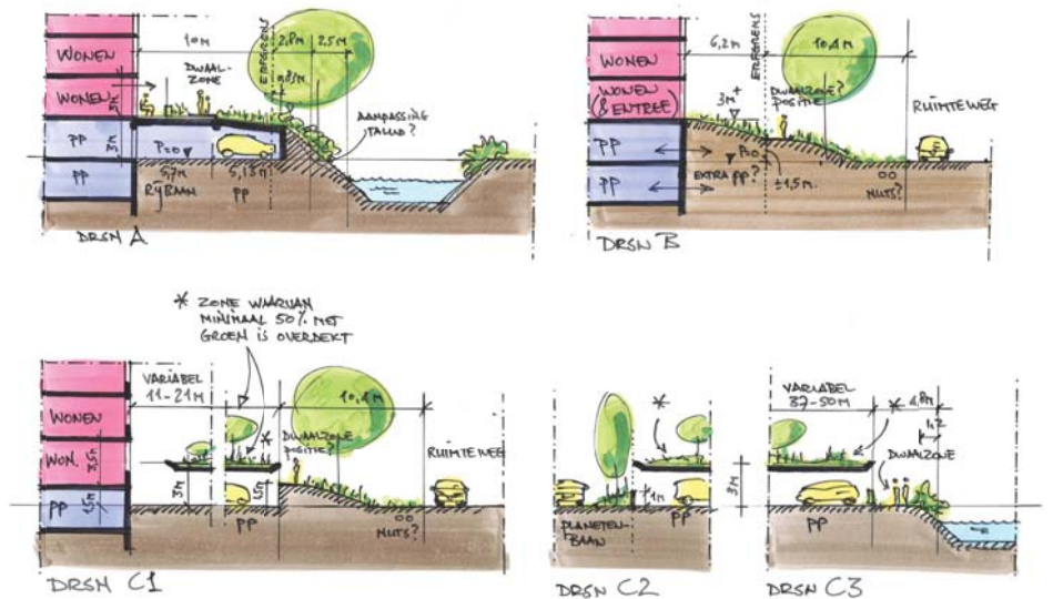
PRINCIPEDOORSNEDEN MAAIVELD CORNER PLAZA - LUNED ARCHITECTEN - 06/04/23
