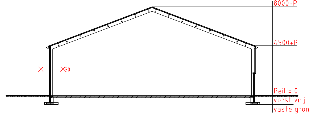
Doorsnede stal L
