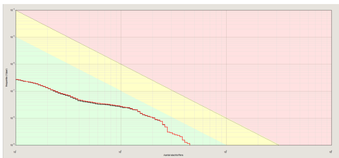
Figuur 7. Groepsrisicocurven
