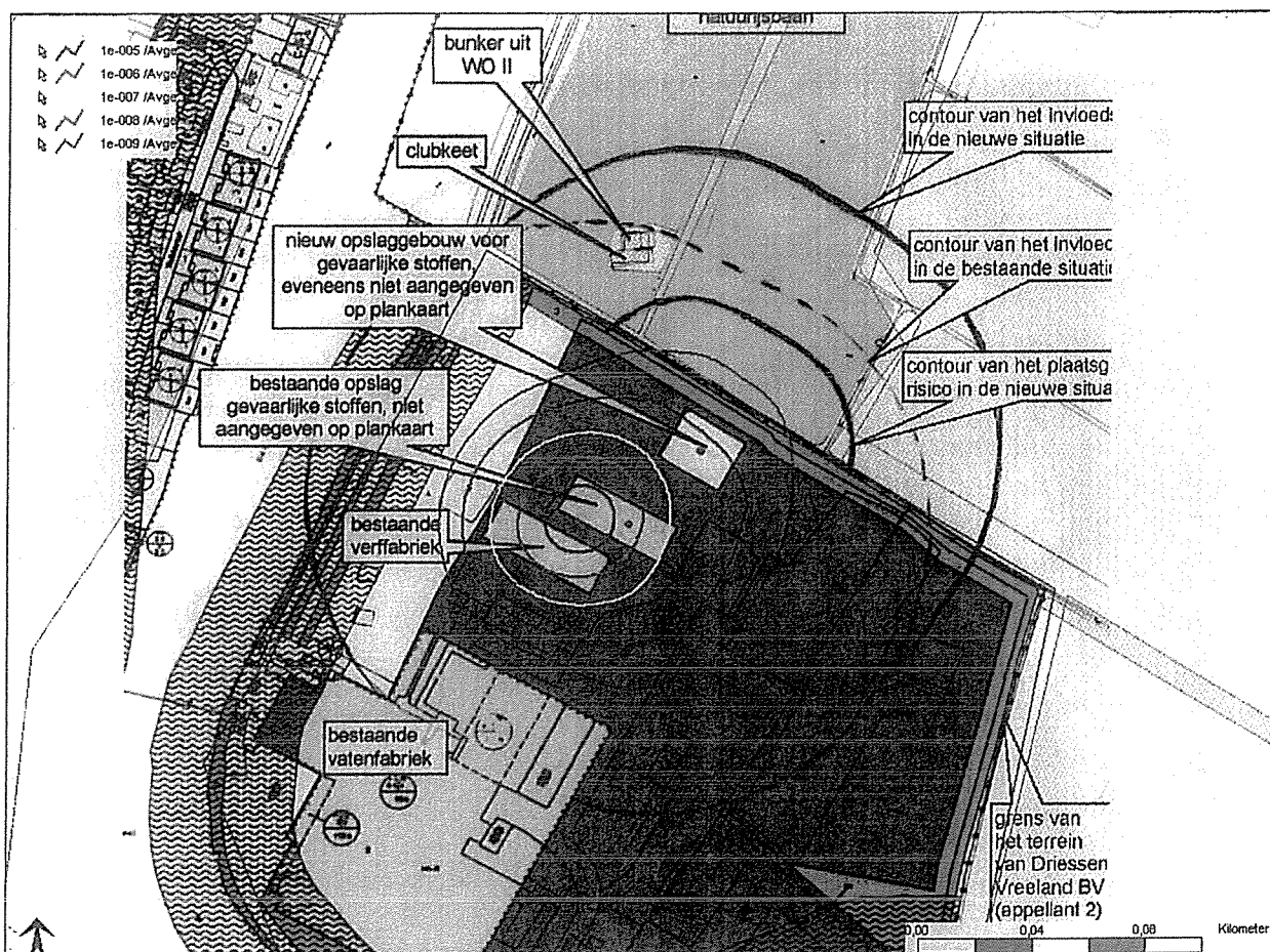
Plaatsgebonden risico contour van PGS 15 loads 22 en 44 en verlading van brandbare vloeistoffen ingetekend op de ondergrond van de provincie.
