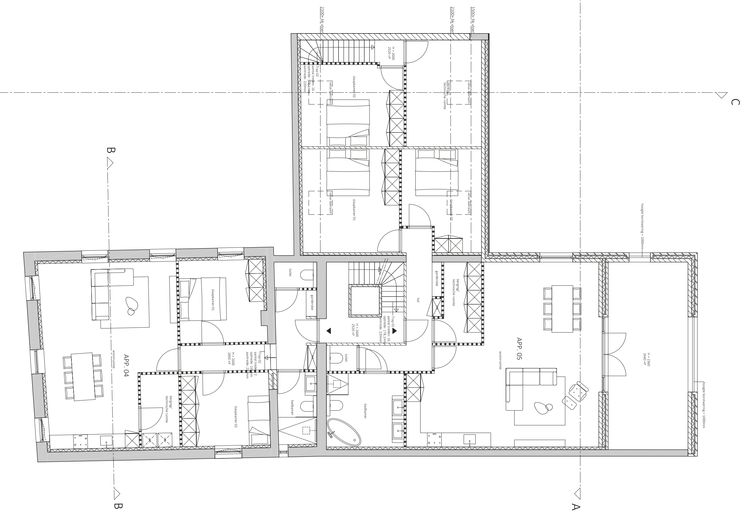
EERSTE VERDIEPING
