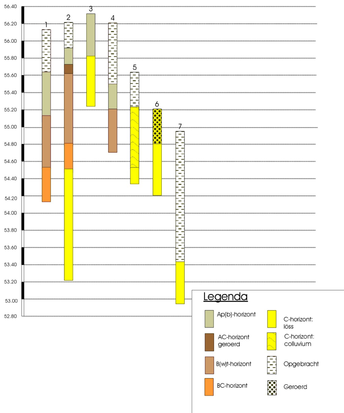
Figuur 20: Boorprofielen
