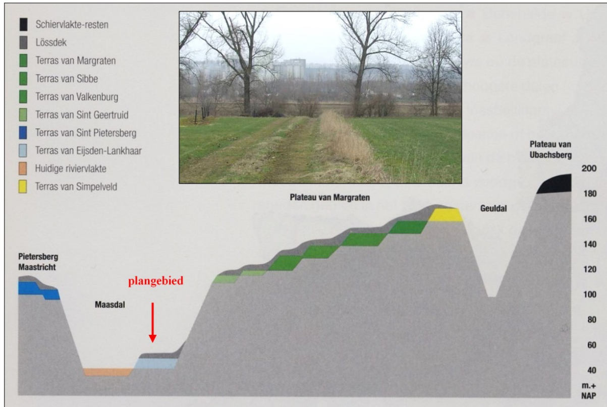
Figuur 7: Schematische weergave van het oost-westprofiel over het huidige Maasdal bij Maastricht en de oudere terrasniveaus (). 11 Het laatglaciale terras van Geistingen wordt hier tot het Maasdal gerekend. Het terras van Mechelen a/d Maas ligt op het niveau van het terras van Eijsden-Lankhaar. De foto-inzet toont de terrasrand gezien van de Schansweg ten zuiden van de bebouwing van Eijsden in westelijke richting met op de achtergrond het huidige Maasdal en daarachter de steile rand van de St. Pietersberg en de groeve van Lixhe.
