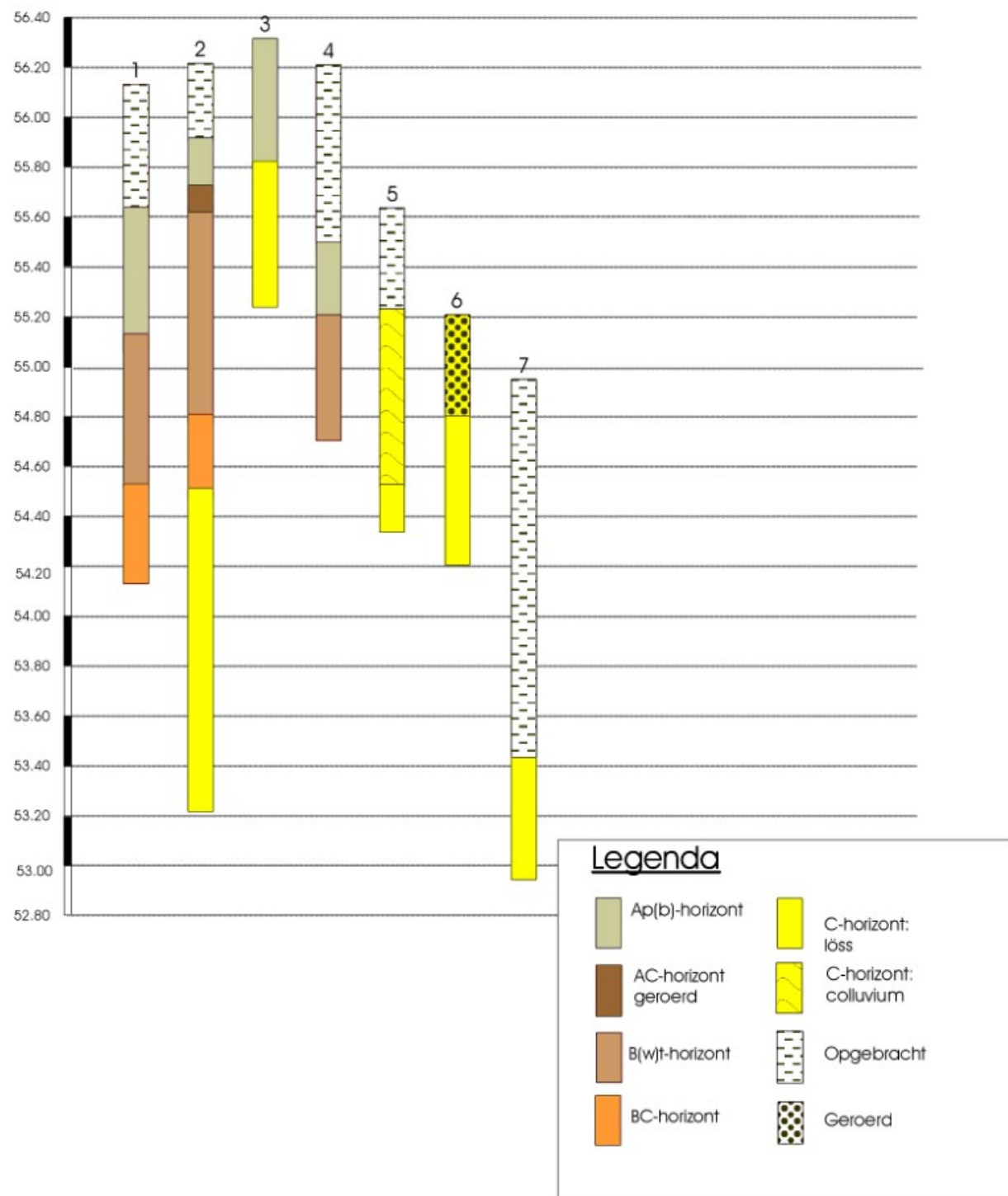
Figuur 20: Boorprofielen
