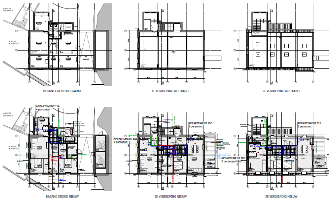
Inrichting hoofdgebouw nieuwe situatie (bron: Vullings de Moor d.d. 18 februari 2020, projectnr. 1882, tekeningnr. OMG-01)
