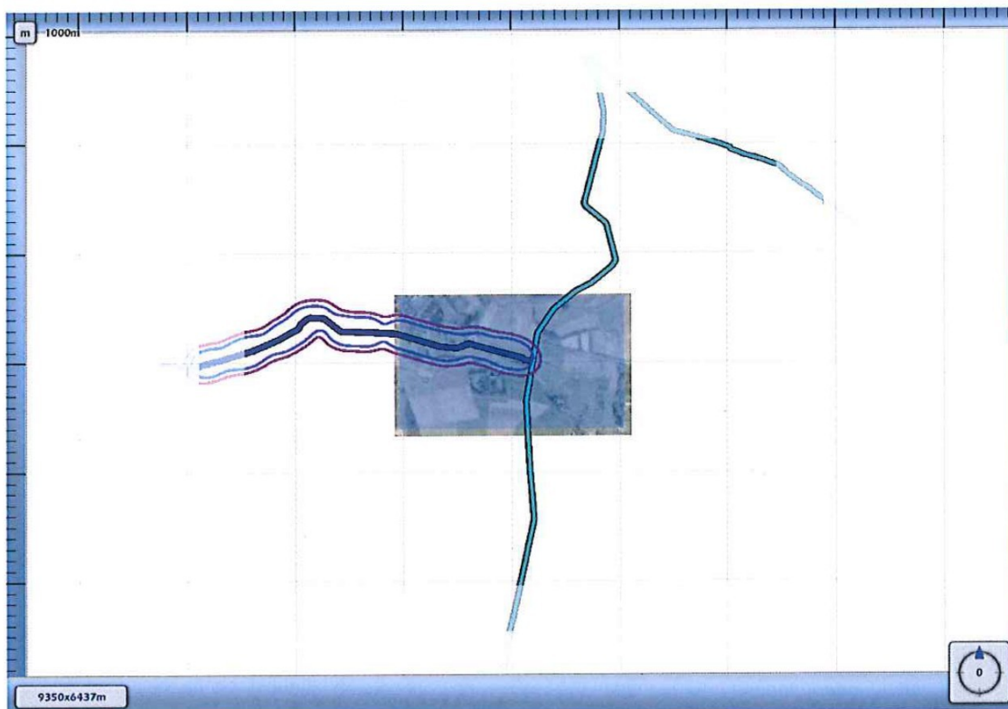
a) Figuur 3.1 Plaatsgebonden risico voor 3492_leiding-A-520-03-deel-1 van N.V. Nederlandse Gasunie
