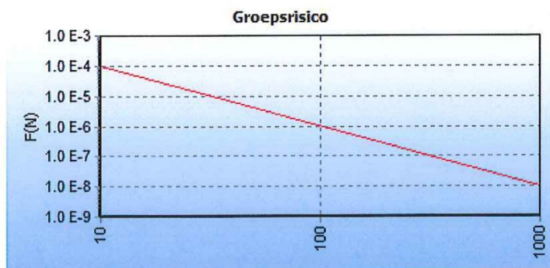
c) Figuur 5.3 FN curve voor 3492_leiding-A-534-deel-1 van N.V. Nederlandse Gasunie voor de kilometer tussen stationing 820.00 en stationing 1820.00
