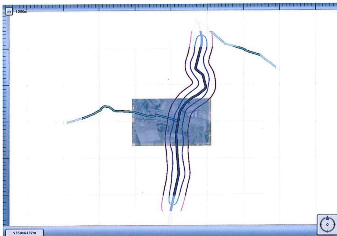
c) Figuur 3.3 Plaatsgebonden risico voor 3492_leiding-A-534-deel-1 van N.V. Nederlandse Gasunie
