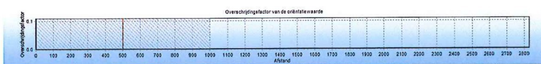
a) Figuur 4.1 Groepsrisico screening voor 3492_leiding-A-520-03-deel-1 van N.V. Nederlandse Gasunie
