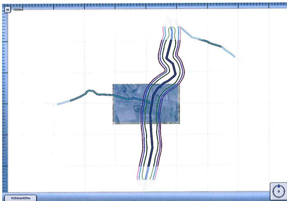
b) Figuur 3.2 Plaatsgebonden risico voor 3492_leiding-A-520-deel-1 van N.V. Nederlandse Gasunie
