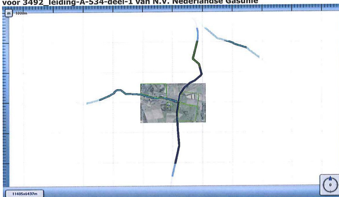
Figuur 4.3 Kilometer leiding behorende bij de maximale overschrijding van de FN-curve voor 3492 leiding-A-534-deel-1 van N.V. Nederlandse Gasunie
