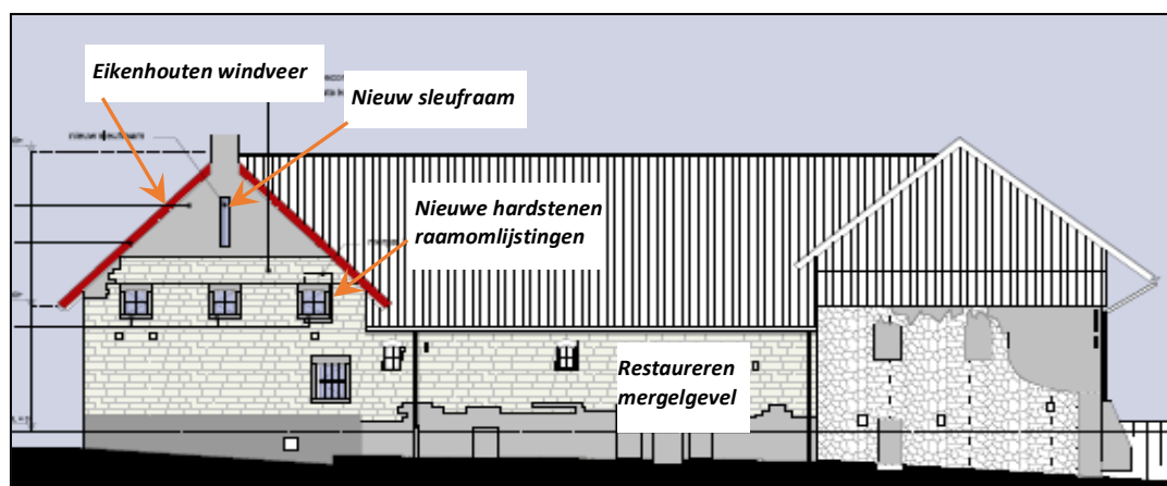
Tekening gevel aan de zijde van de Dorpsstraat
