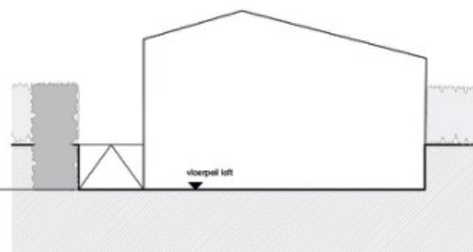
principe dwarsdoorsnede i.r.t. aanwezig reliëf (ter hoogte van hagen/hogstamfruitboomgaard)
