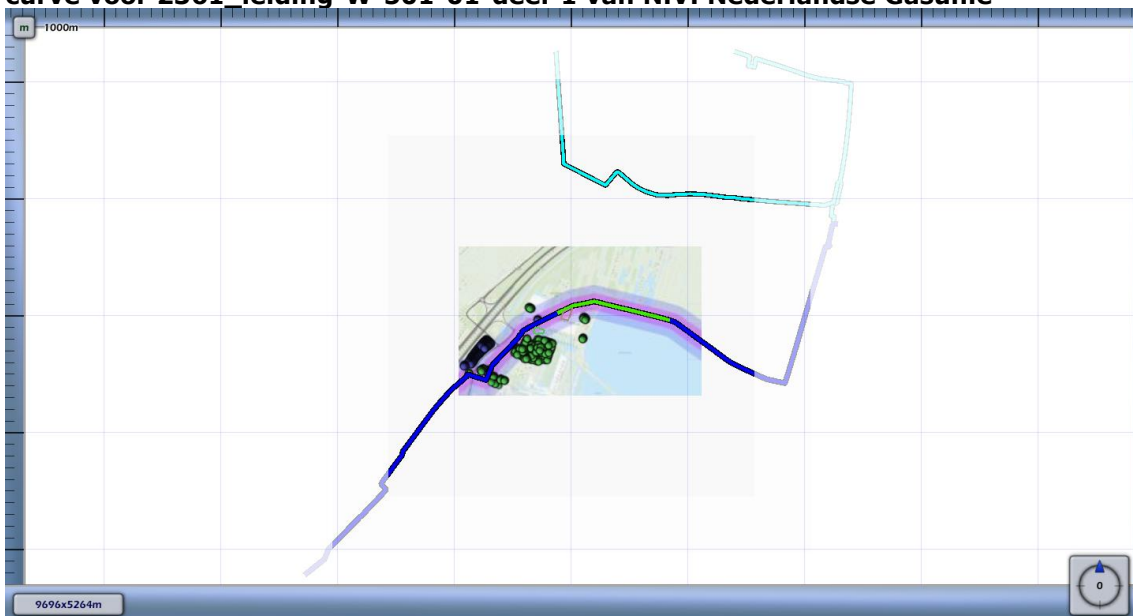
Figuur 4.2 Kilometer leiding behorende bij de maximale overschrijding van de FN-curve voor 2361_leiding-W-501-01-deel-1 van N.V. Nederlandse Gasunie
