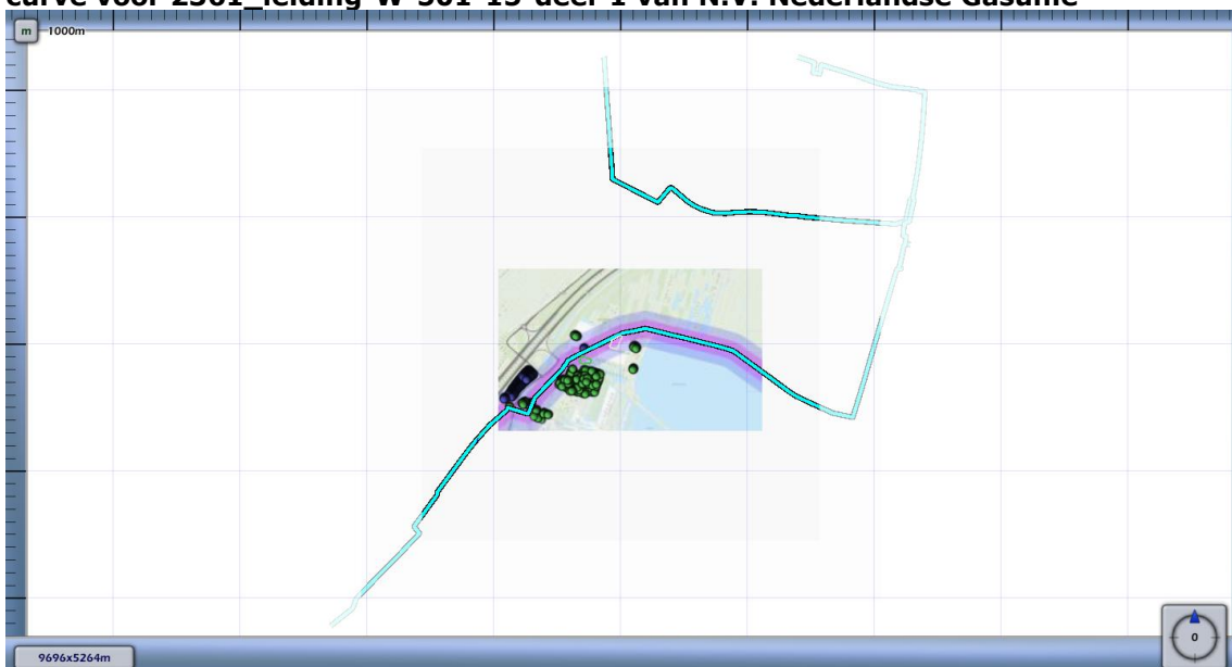
Figuur 4.4 Kilometer leiding behorende bij de maximale overschrijding van de FN-curve voor 2361_leiding-W-501-15-deel-1 van N.V. Nederlandse Gasunie
