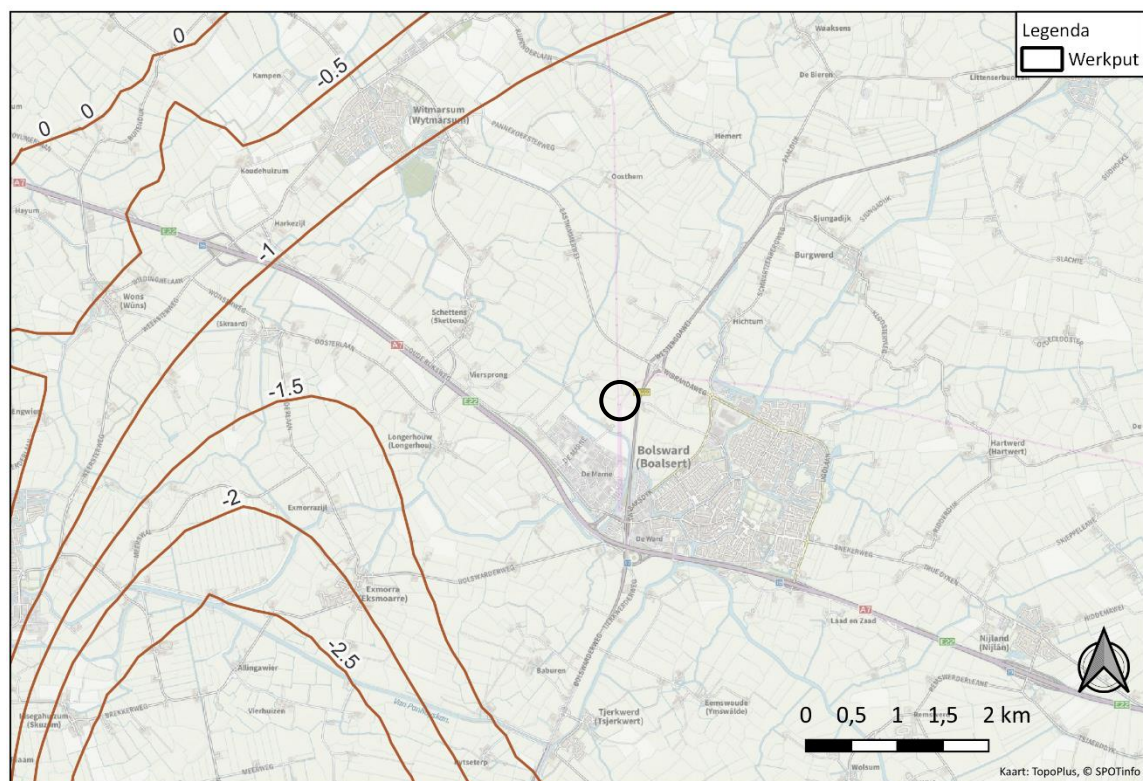
Figuur 2.3 Ligging isohypsen eerste watervoerende pakket ten opzichte van de werklocatie. Bron: TNO.
