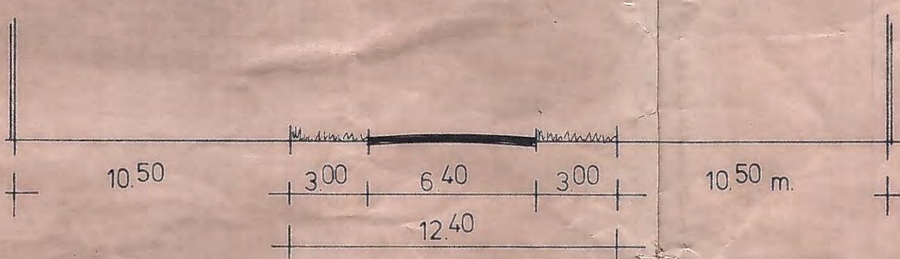
DWARSPROFIEL (RONDWEG HEEMELUM) schaal 1:200
