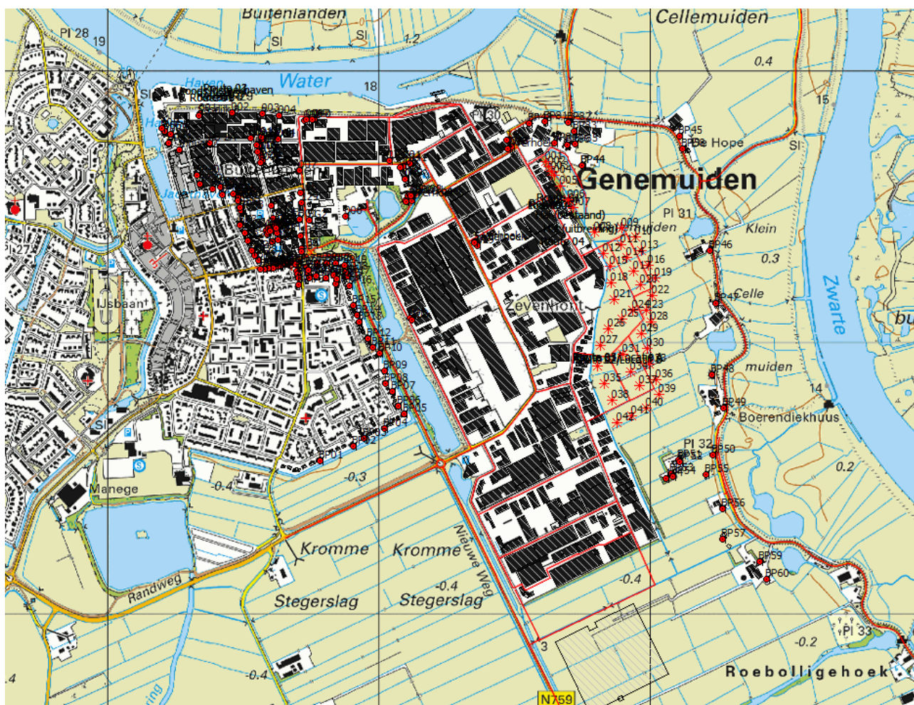
Afbeelding 4: rekenmodel
