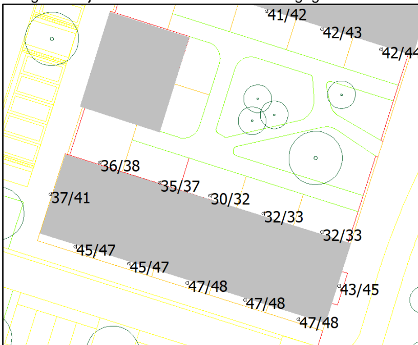
Figuur 9, berekende waarde met scherm
