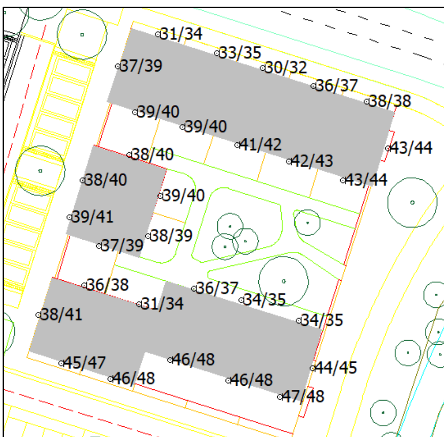
Figuur 10, versprongen bouwblok
