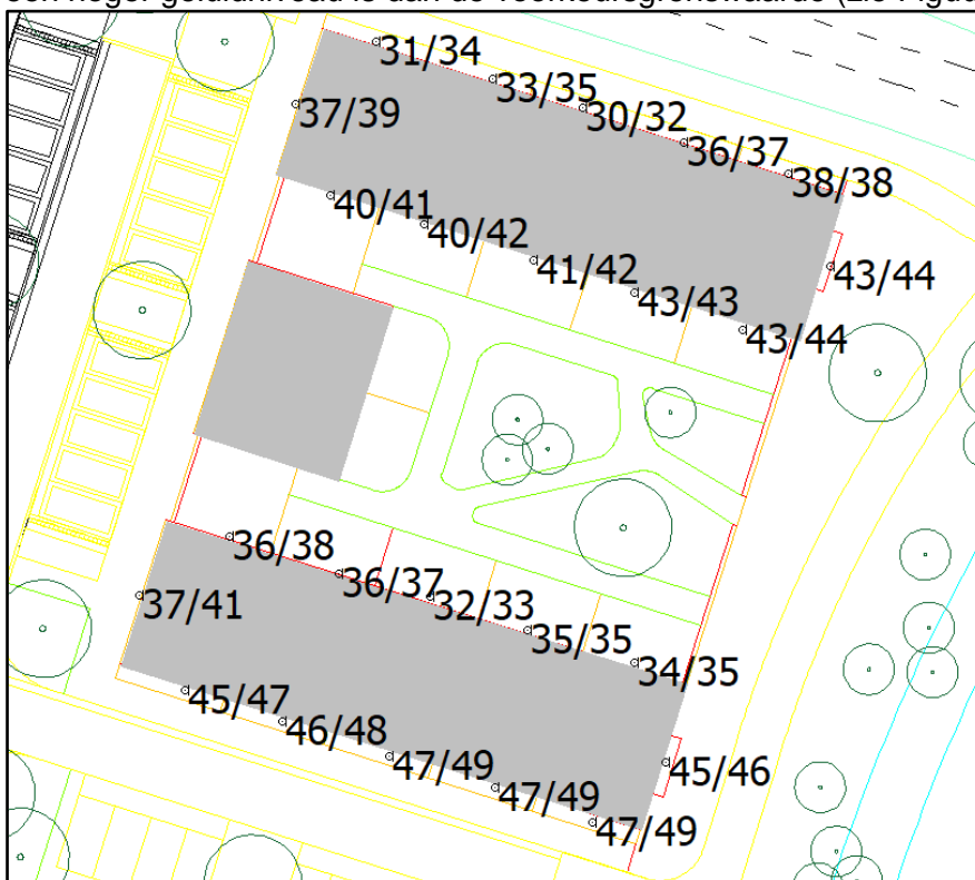
Figuur 6, geluidbelasting met verplaatst 50 km/uur bord
