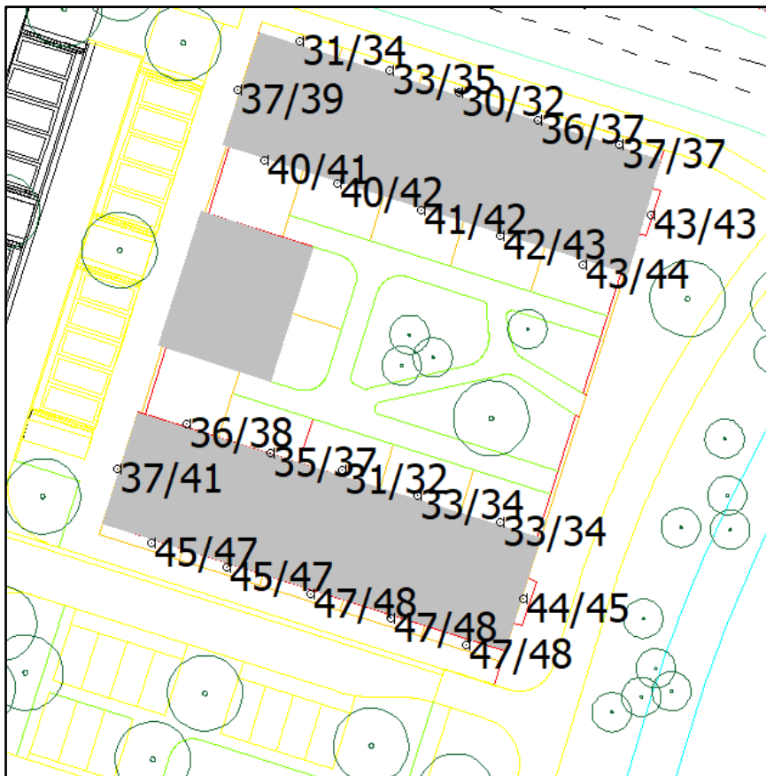
Figuur 7, geluidbelasting met dunne deklaag A en 50 km/uur
