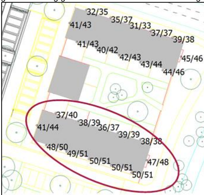
Figuur 4, geluidbelasting zuidelijke bouwblok
