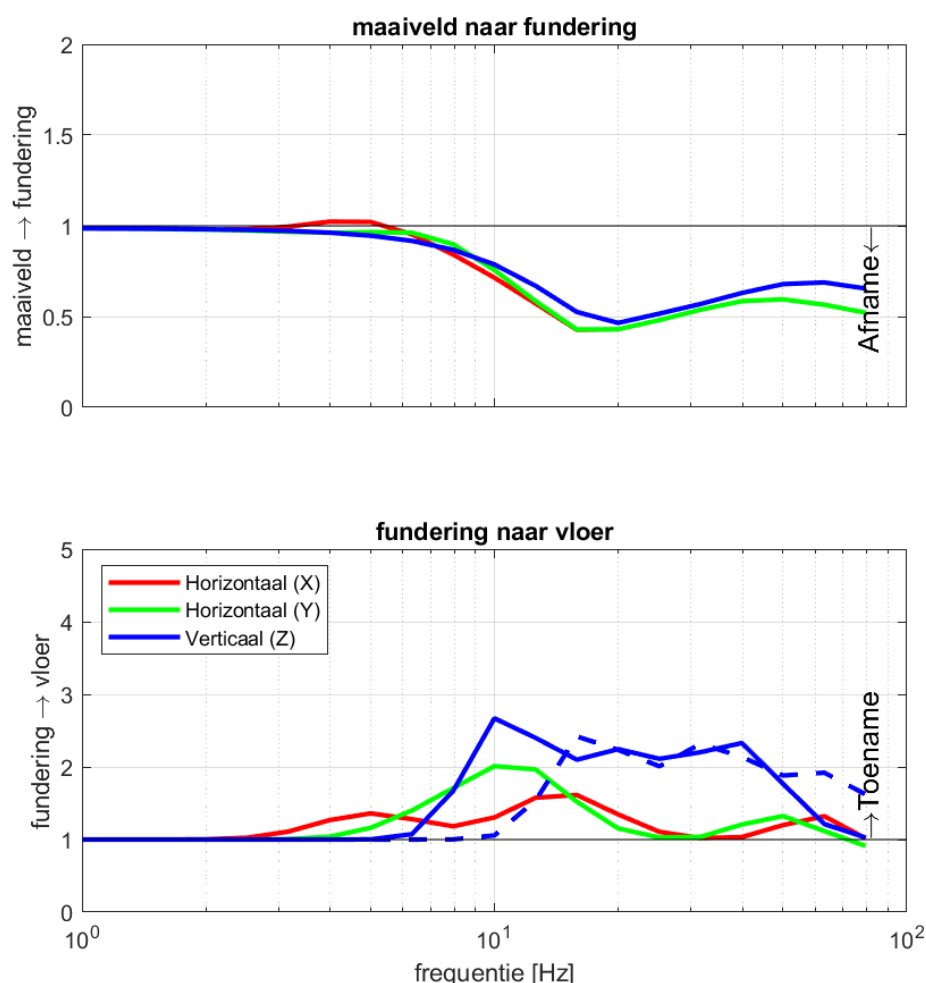
Figuur 10 Buildyn-resultaten voor een vrijstaande woning van 12 x 8 meter grondvlak, 6 meter bouwhoogte en een kanaalplaatvloer van 200 mm, casco van kalkzandsteen en metselwerk
