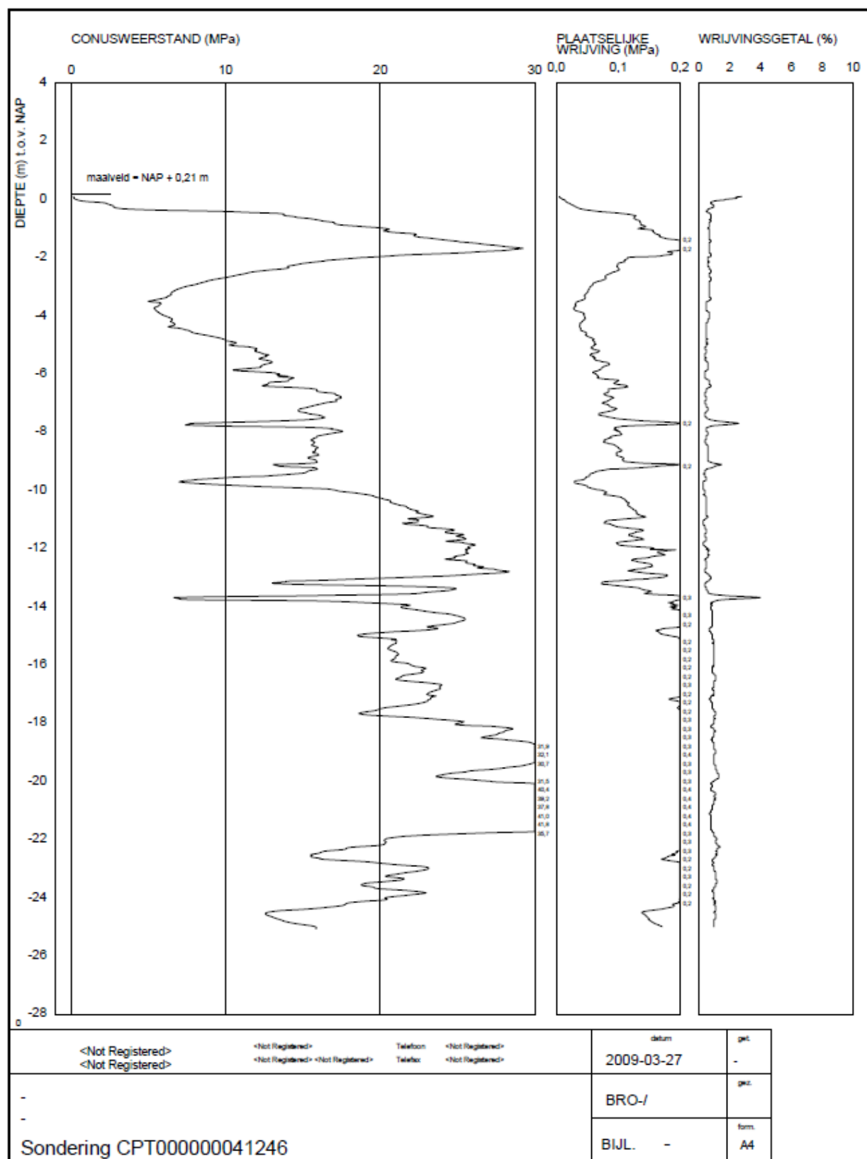
Figuur 8 Sondering nabij het onderzoeksgebied, CPT000000041246
