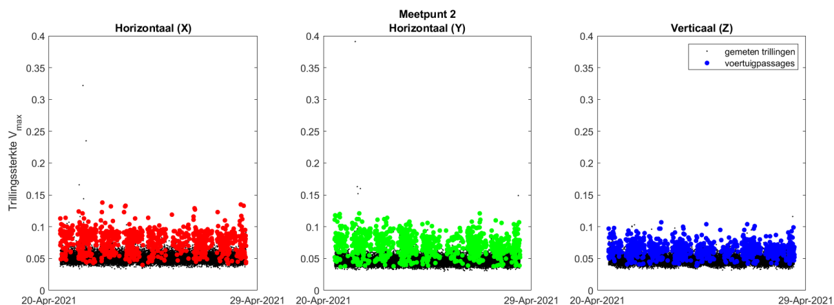
Figuur 12 Gemeten trillingen bij meetpunt 2 (maaiveld, noordzijde perceel)
