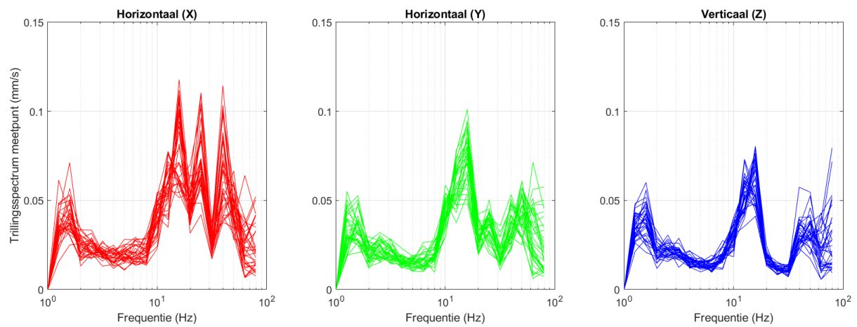
Figuur 14 Tertsbandspectra bij meetpunt 2
