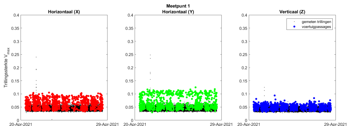
Figuur 11 Gemeten trillingen bij meetpunt 1 (maaiveld, zuidzijde perceel)
