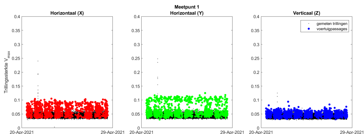
Figuur 6 Gemeten trillingen op maaiveld
