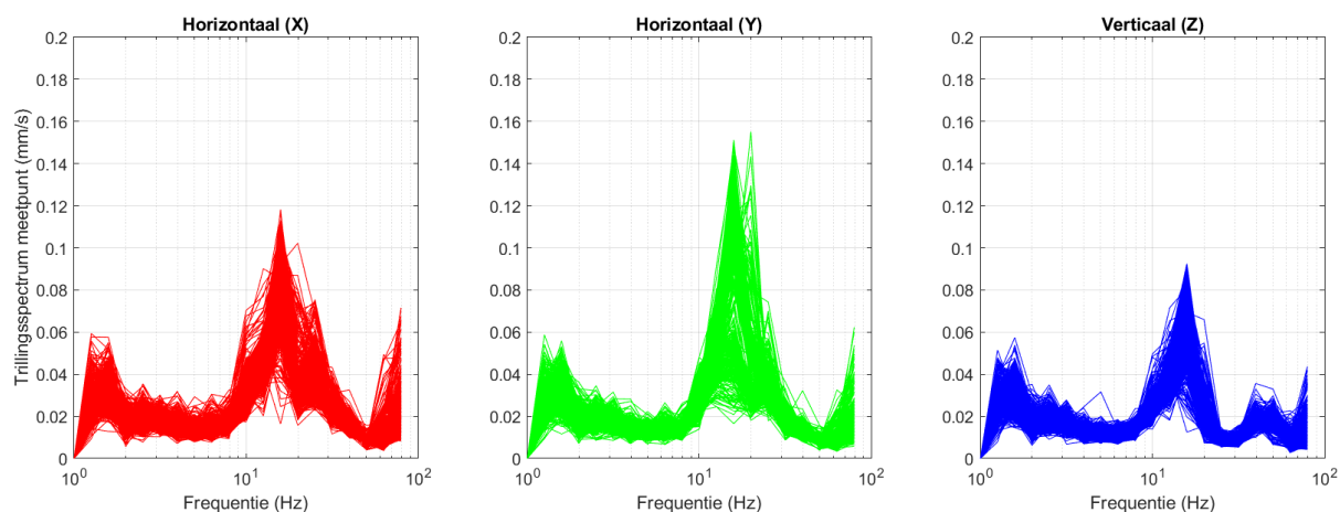
Figuur 13 Tertsbandspectra bij meetpunt 1
