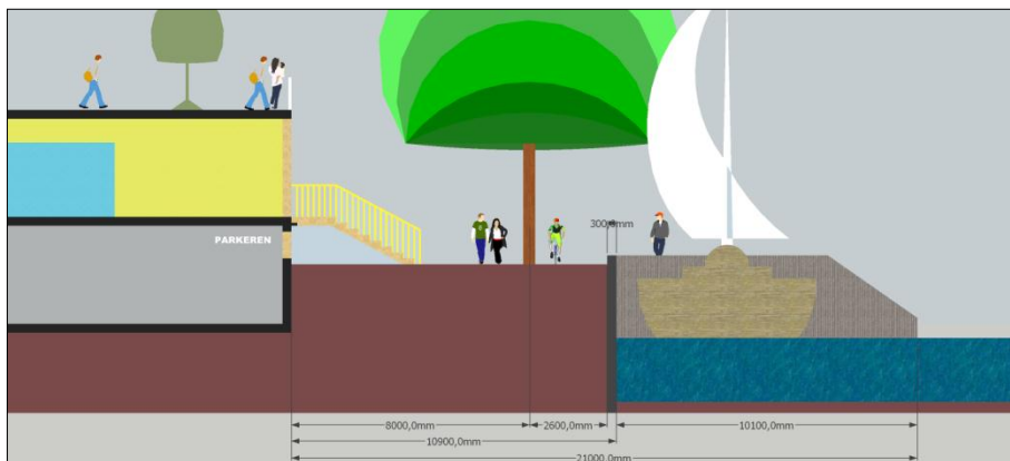
Principeprofiel wandelkade Rensel
