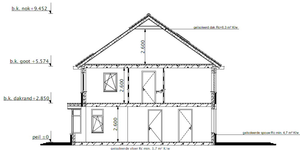
doorsnede A-A
