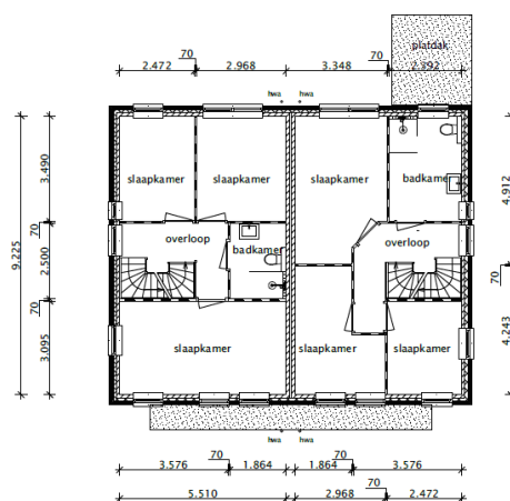
plattegrond Verdieping
