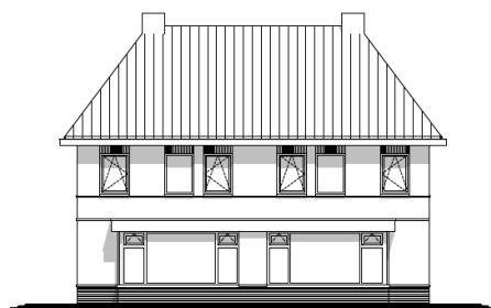
aanzicht Voorgevel
