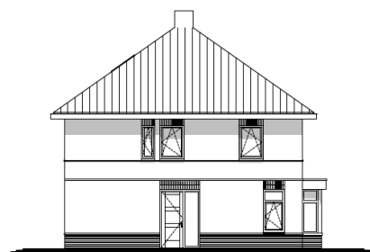
aanzicht Linkerzijgevel
