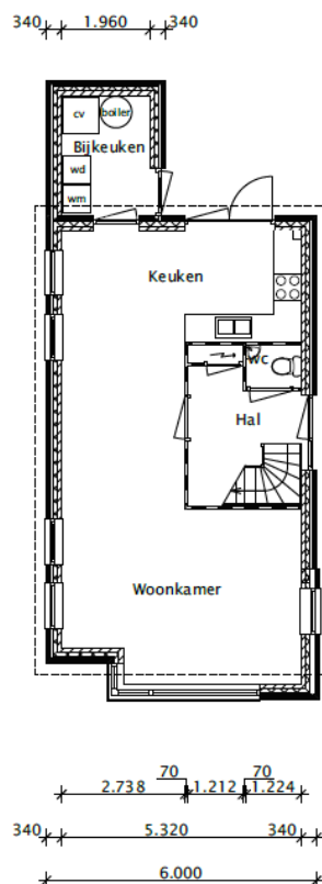
plattegrond Beganegrond
