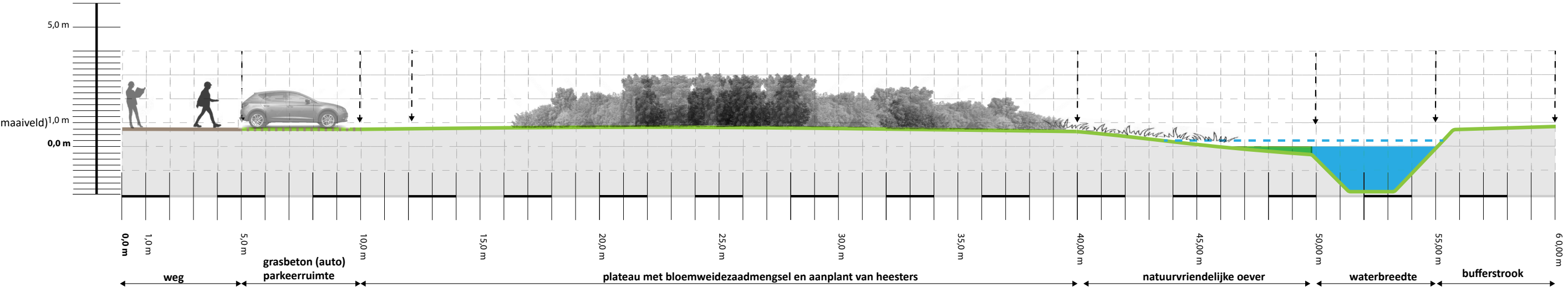
Doorsnede 2 door parkeerplaats, plateau met struikbeplanting en sloot met brede natuurvriendelijke oever
