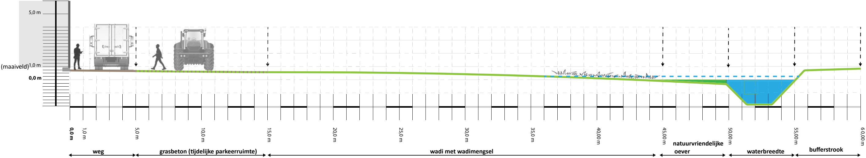
Doorsnede 1 wadi en sloot
