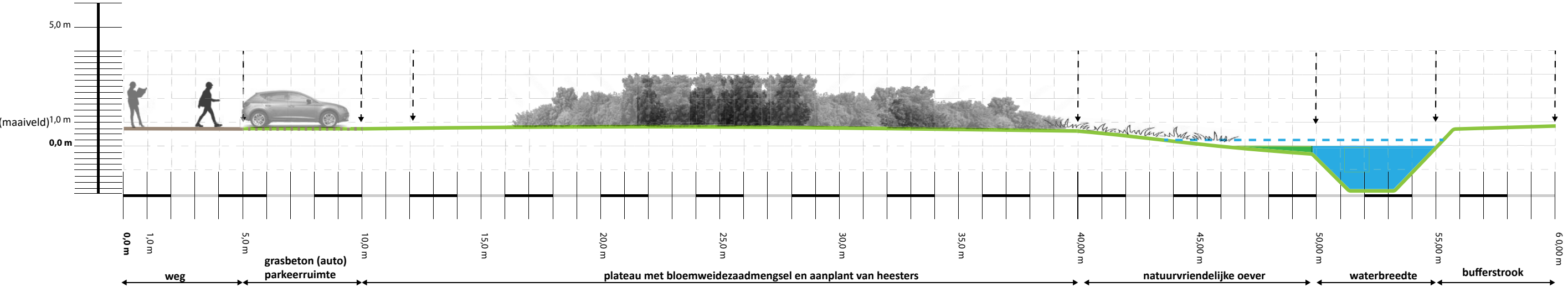
Doorsnede 2 parkeerplaats, plateau met struikbeplanting en sloot met brede natuurvriendelijke oever
