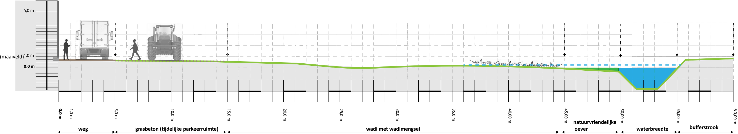
Doorsnede 1 door het wadi-gebied en de sloot
