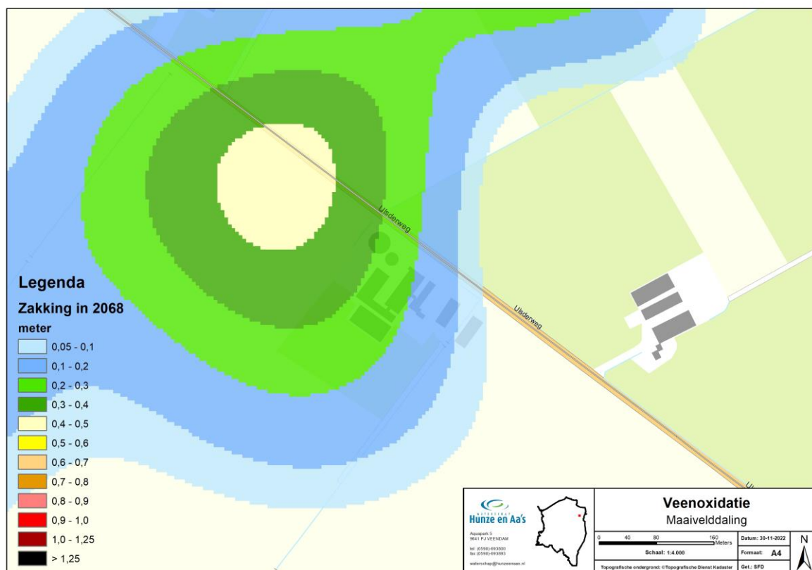
Figuur 2: Prognose maaiveld daling in 2068 als gevolg van autonome veenoxidatie
