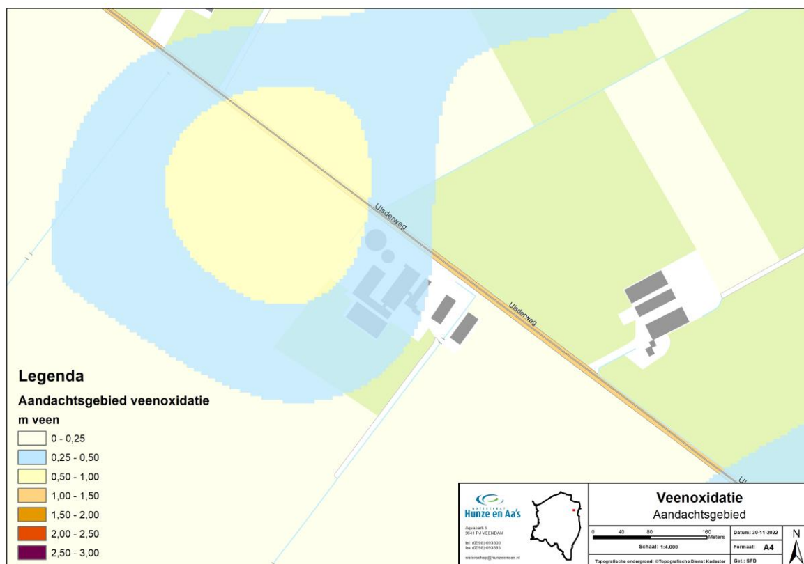
Figuur 1: aandachtgebied veenoxidatie (veendikte boven GLG (gemiddeld laagste grondwaterstand) en 1m daaronder)
