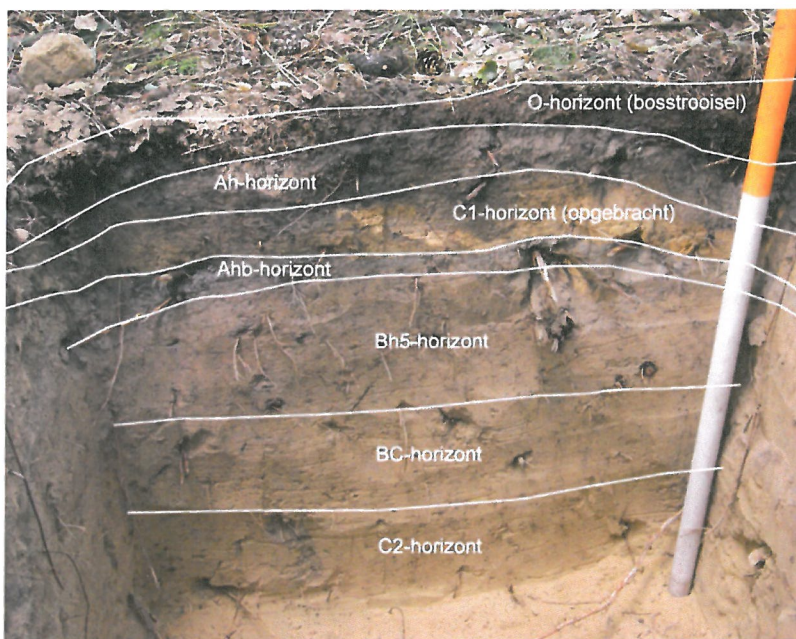
Putprofiel C: maaiveldhoogte 35,93 m +NAP
