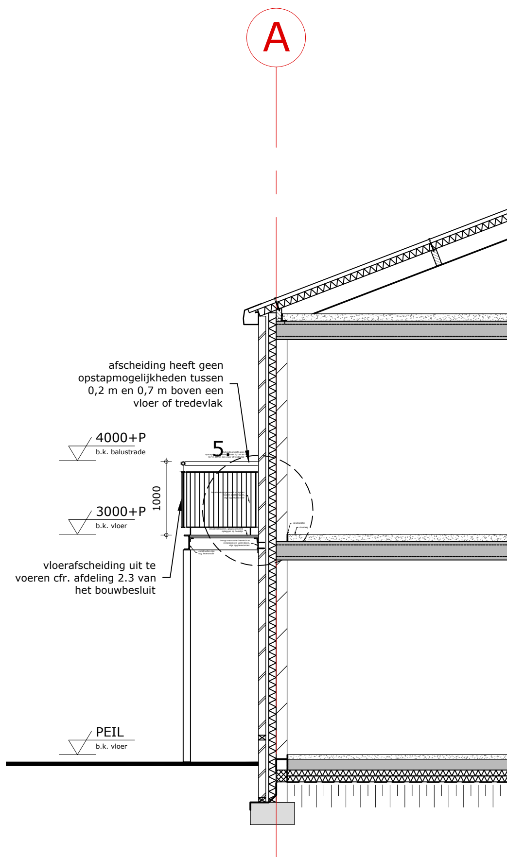
doorsnede B-B (schaal 1:50)
