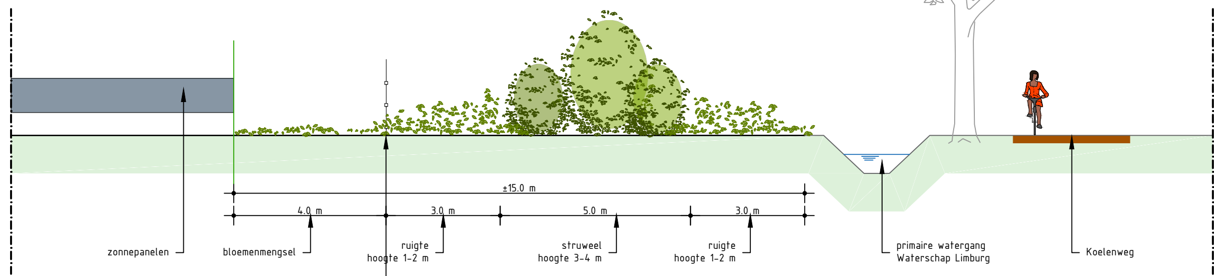
DOORSNEDE A-A Schaal 1:100
