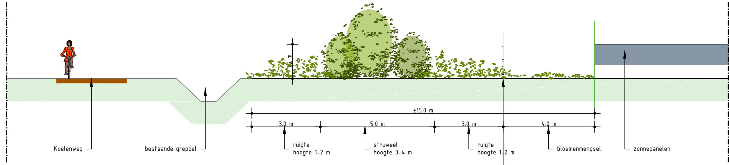
DOORSNEDE B-B Schaal 1:100
