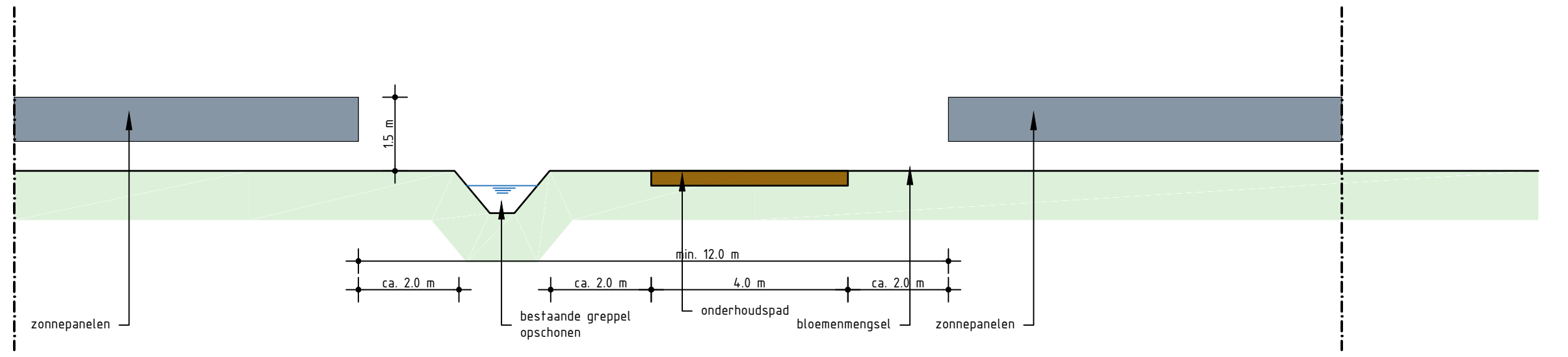
DOORSNEDE C-C Schaal 1:100
