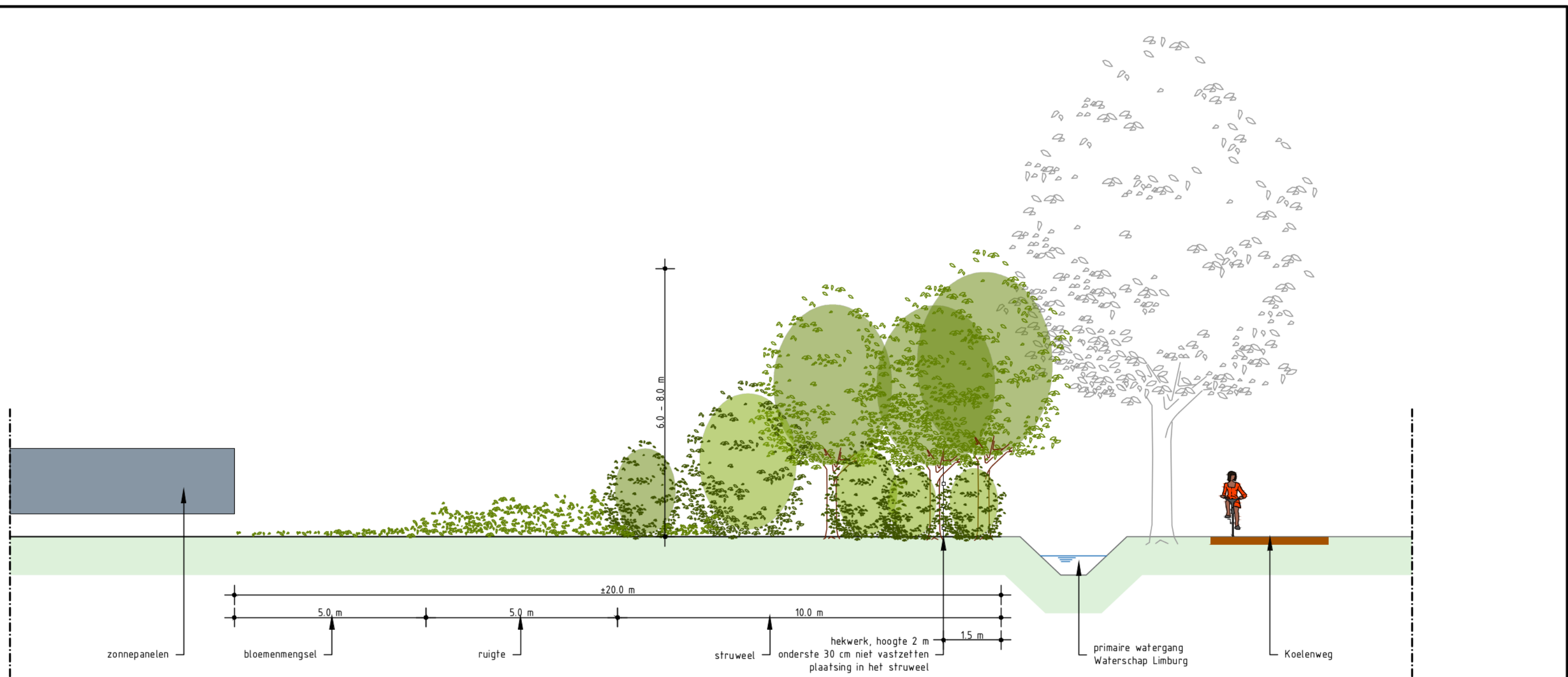
DOORSNEDE A-A Schaal 1:100
