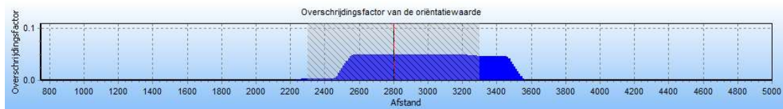
Afbeelding 3 Groepsrisico screening A-520-01-deel-1 huidige situatie ter hoogte van het plangebied
