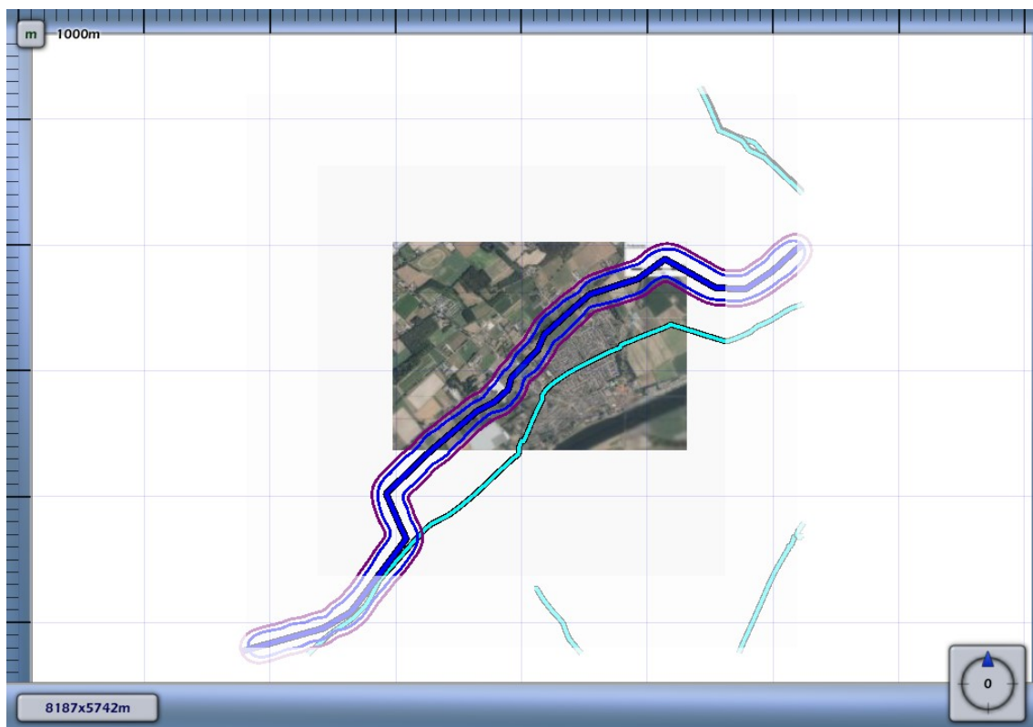
3.1 Figuur 3.1 Plaatsgebonden risico voor 7023_leiding-A-520-01-deel-1 van N.V. Nederlandse Gasunie
