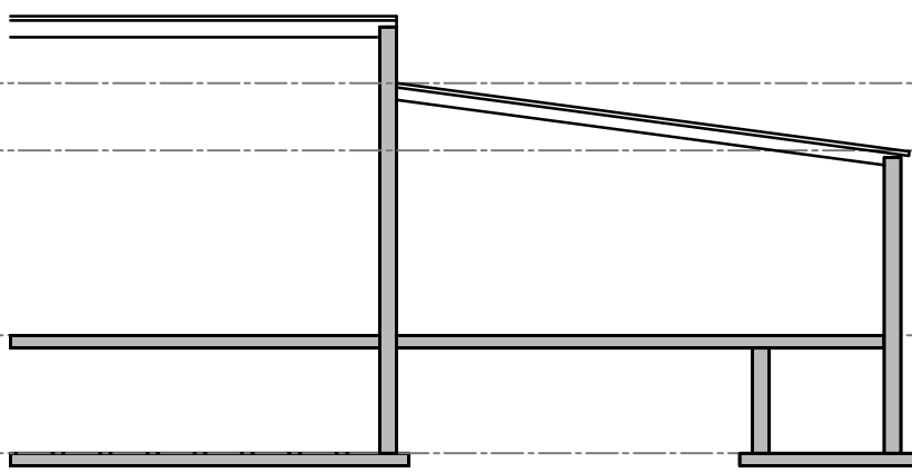
doorsnede stal A - ( A2-A2)
