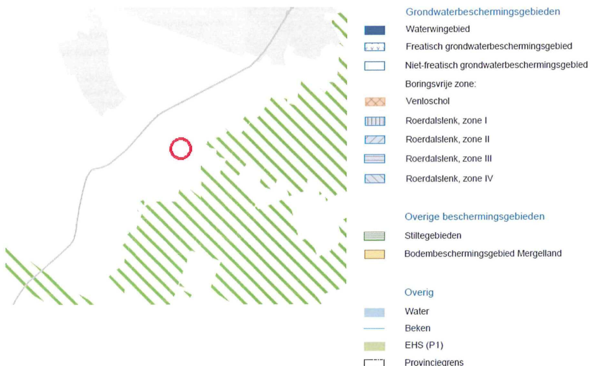
afbeelding 8: Grondwaterbeschermingszones
