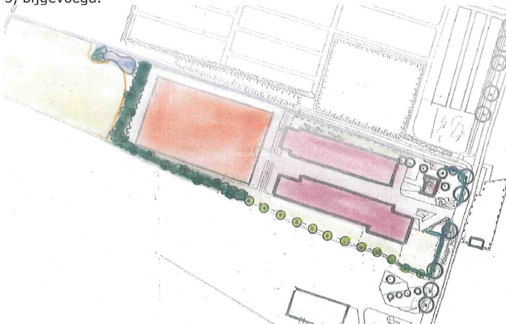
afbeelding 12, landschappelijke inpassing
