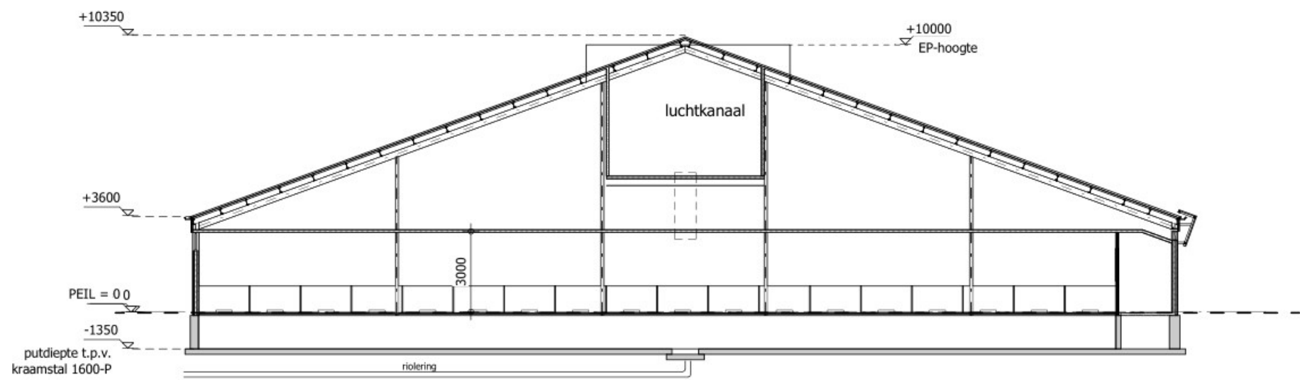
DOORSNEDE GEBOUW 1
