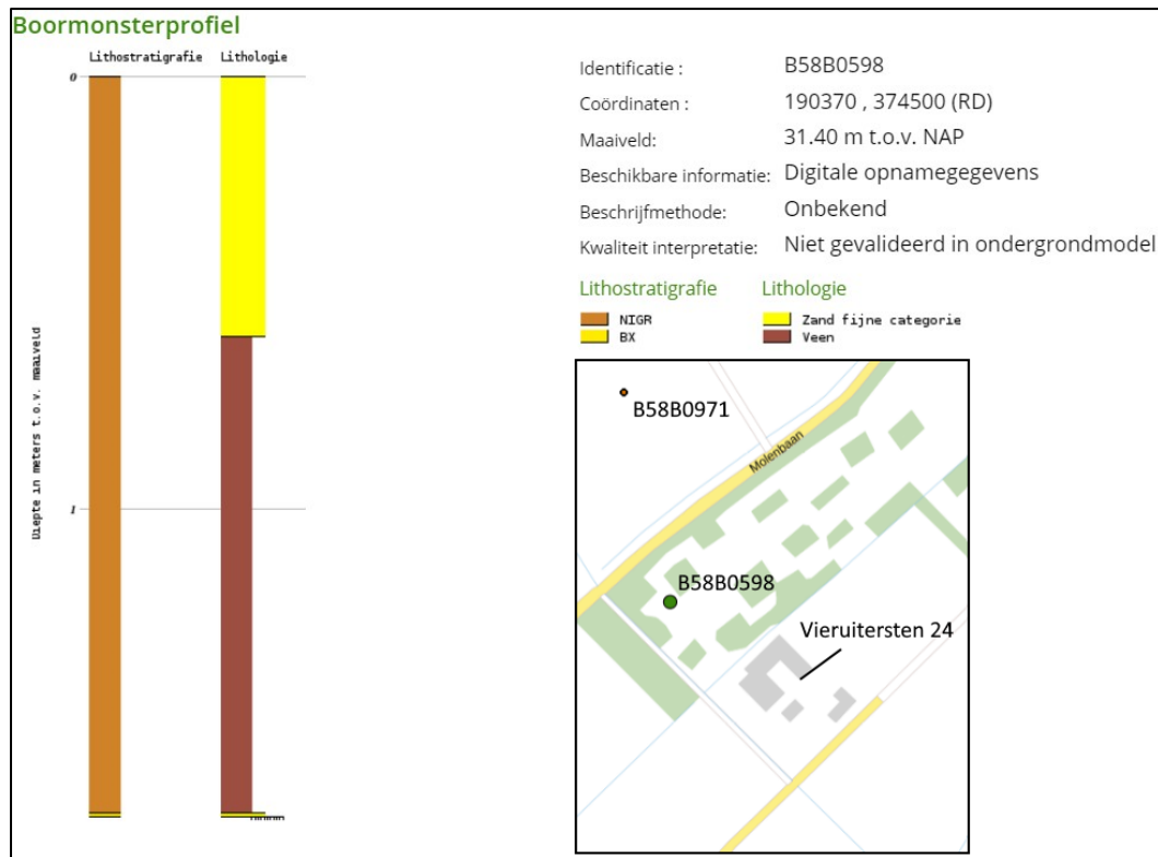
Figuur 3: Boorstaat van boring B58B0598. De locatie van B58B0971 is ook gegeven, en bevat geen veen enkel matig fijn en matig grof zand. BRON: DINOLOket
