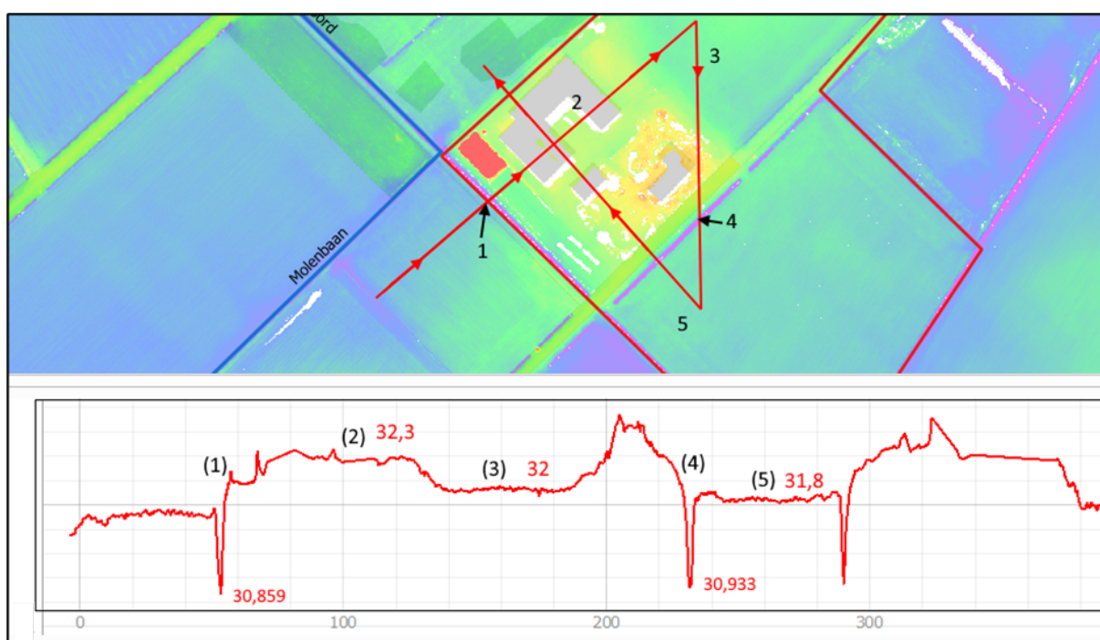
Figuur 5: Hoogteverloop omgeving met ingesneden sloten aldus AHN4. Langs de doorsnede zijn waarden gegeven in meter NAP. Het AHN4 meet niet beneden het waterniveau; het niveau is de laagste meting boven het waterpeil en is hierdoor een redelijke aanname van het peil in de watergang
