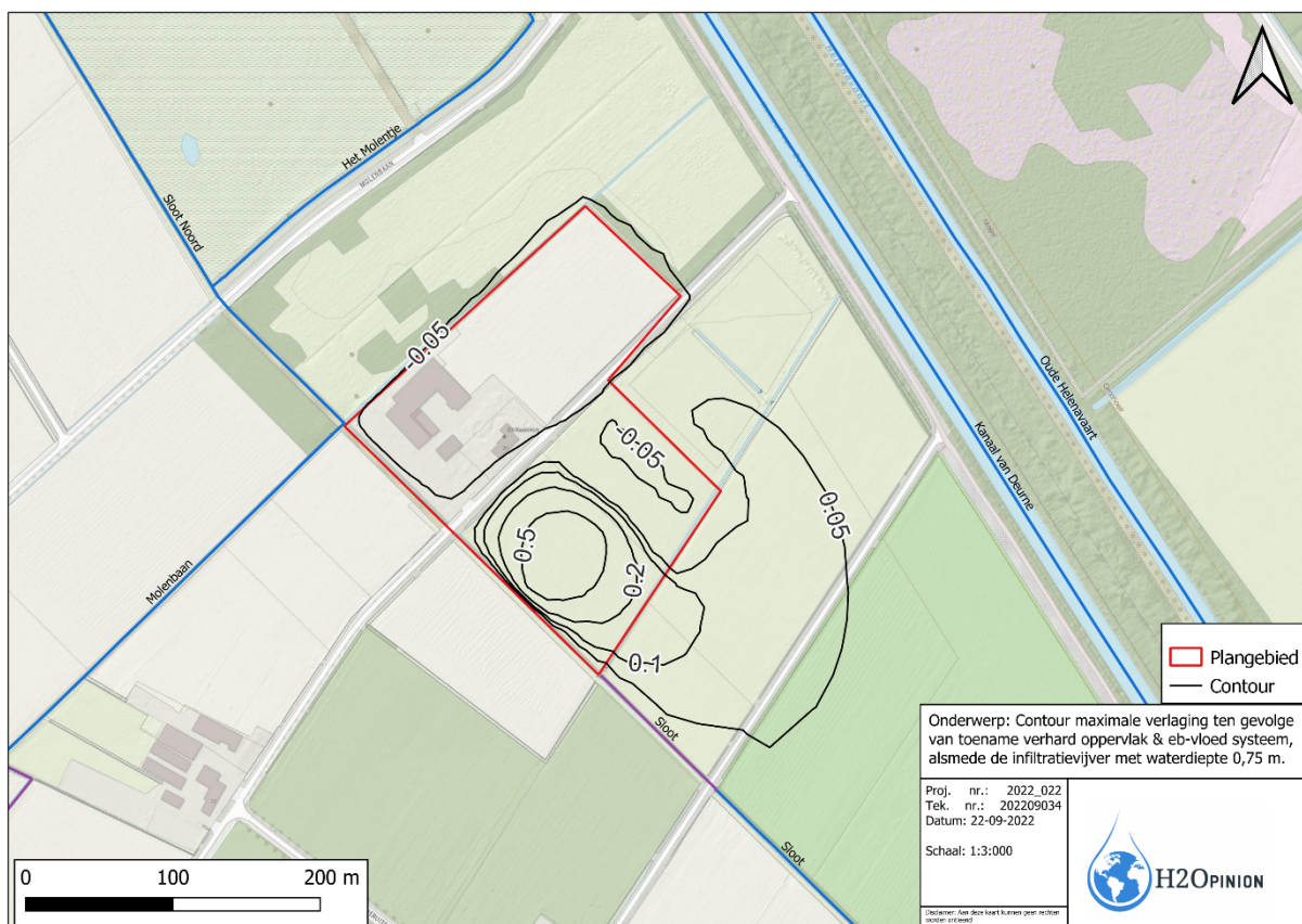
Figuur 2: Invloed bebouwing en infiltratievrijer op de grondwaterstanden in de omgeving volgens de MicroFEM modellering
