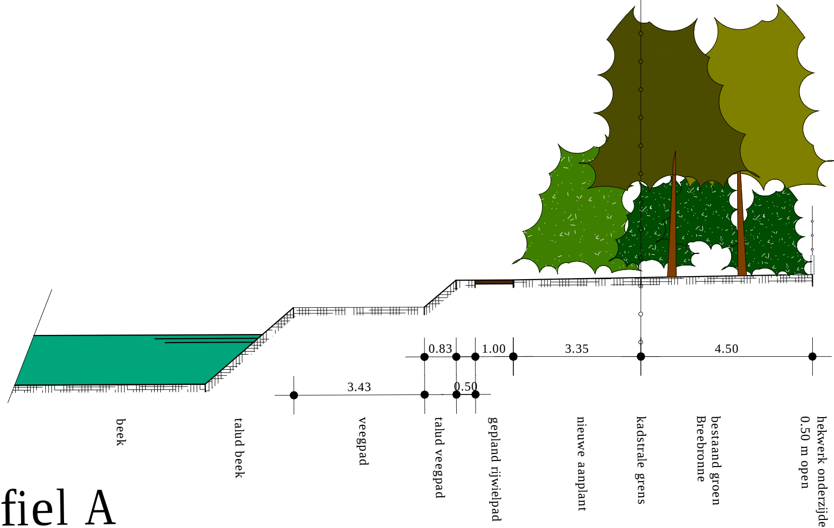
Dwarsprofiel A schaal 1:100
