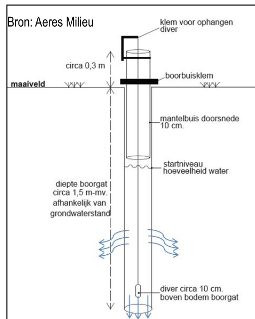
Afbeelding 6: Principetekening Porchetest
