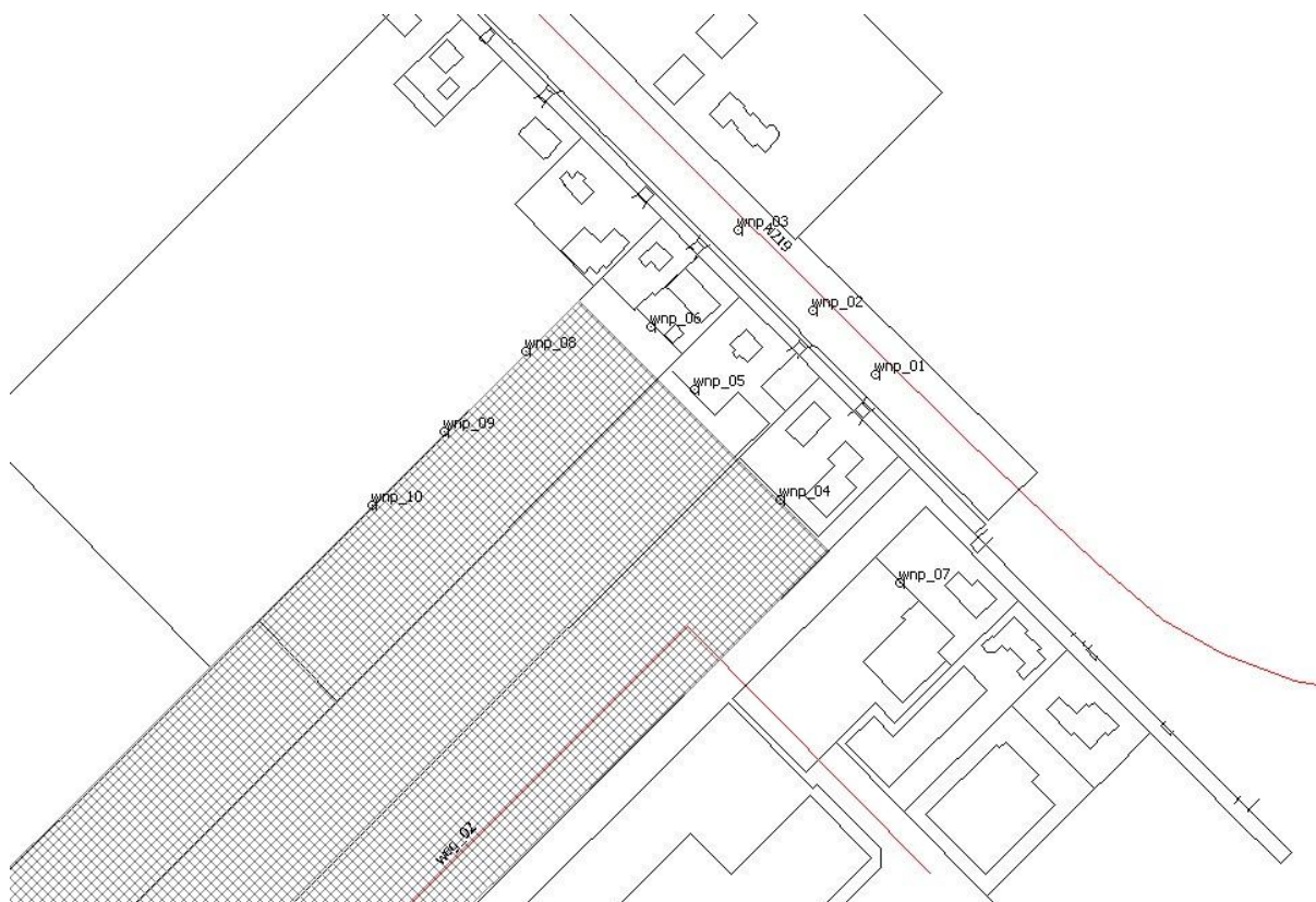
Figuur 5.4.1: Overzicht gehanteerd immissiepunten
