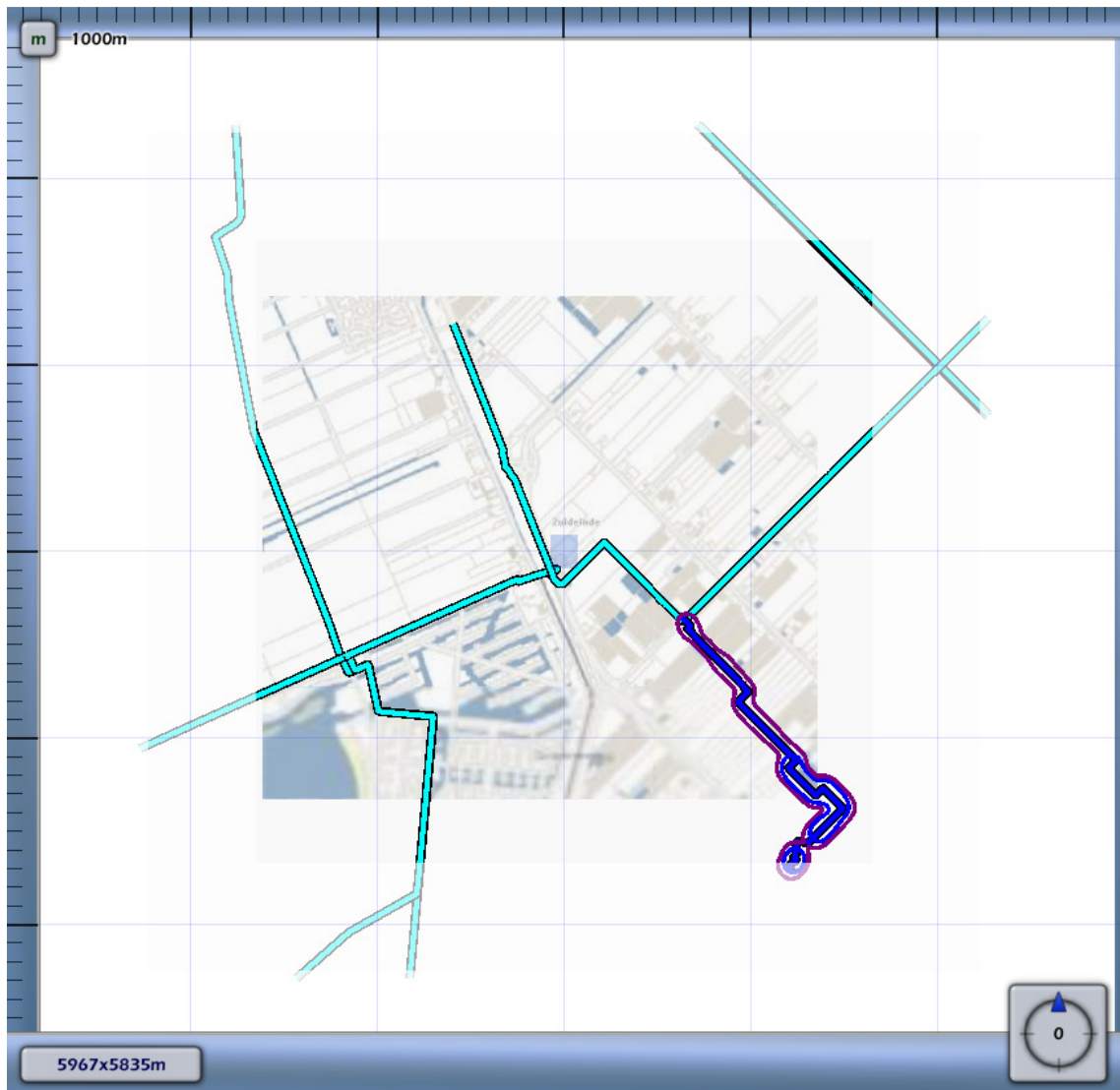
3.10 Figuur 3.10 Plaatsgebonden risico voor 398_leiding-W-521-29-deel-1 van N.V. Nederlandse Gasunie
