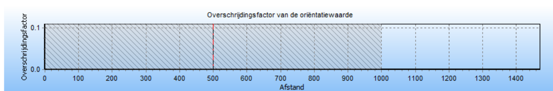
4.8 Figuur 4.8 Groepsrisico screening voor 398_leiding-W-521-04-deel-1 van N.V. Nederlandse Gasunie
