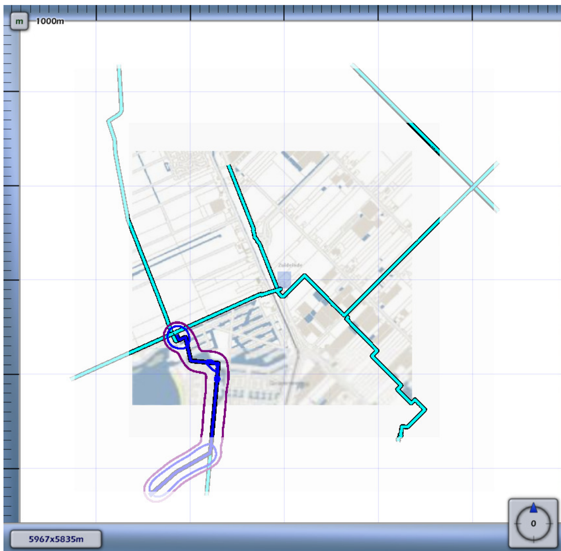
3.8 Figuur 3.8 Plaatsgebonden risico voor 398_leiding-W-521-04-deel-1 van N.V. Nederlandse Gasunie
