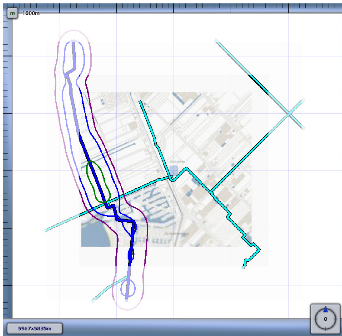
3.1 Figuur 3.1 Plaatsgebonden risico voor 398_leiding-A-518-deel-1 van N.V. Nederlandse Gasunie
