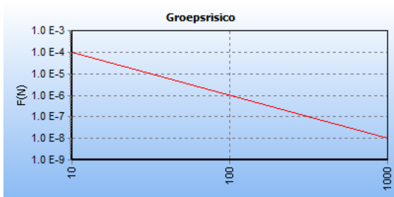
5.10 Figuur 5.10 FN curve voor 398_leiding-W-521-29-deel-1 van N.V. Nederlandse Gasunie voor de kilometer tussen stationing 0.00 en stationing 1000.00
