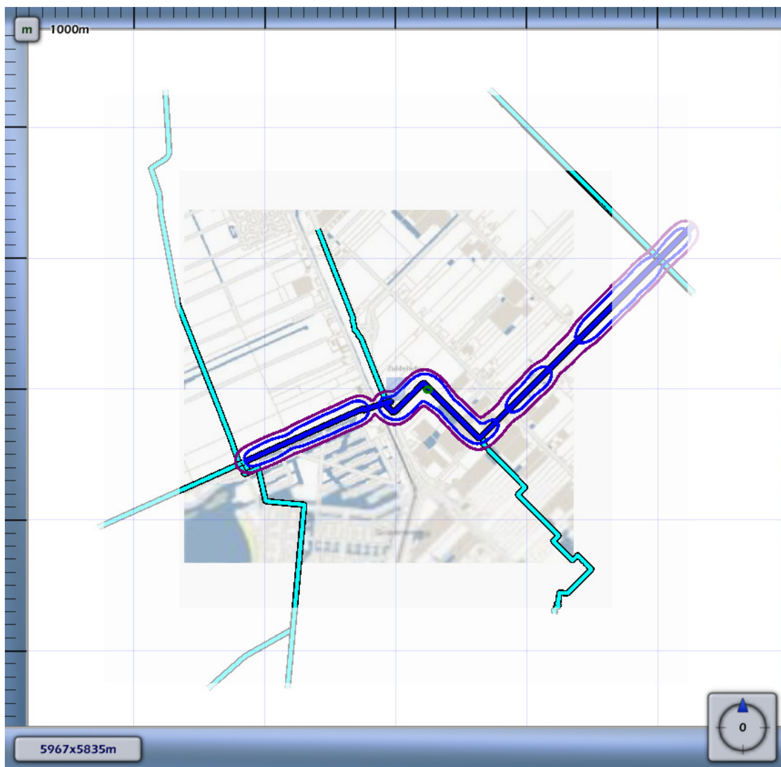
3.7 Figuur 3.7 Plaatsgebonden risico voor 398_leiding-W-521-01-deel-4 van N.V. Nederlandse Gasunie
