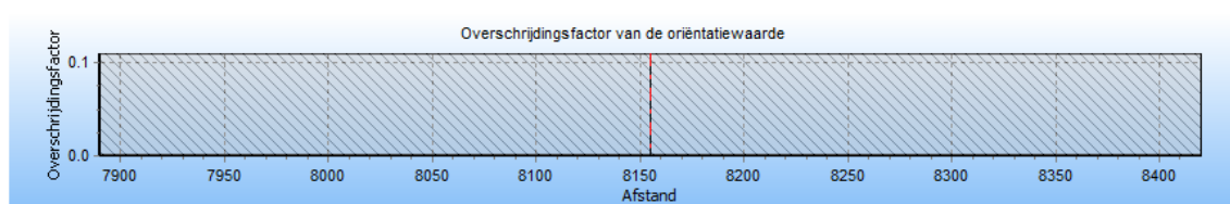
4.5 Figuur 4.5 Groepsrisico screening voor 398_leiding-W-521-01-deel-2 van N.V. Nederlandse Gasunie
