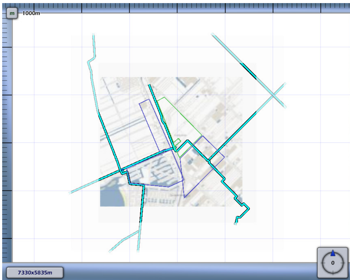
4.5 Figuur 4.5 Groepsrisico screening voor 398_leiding-W-521-01-deel-2 van N.V. Nederlandse Gasunie
