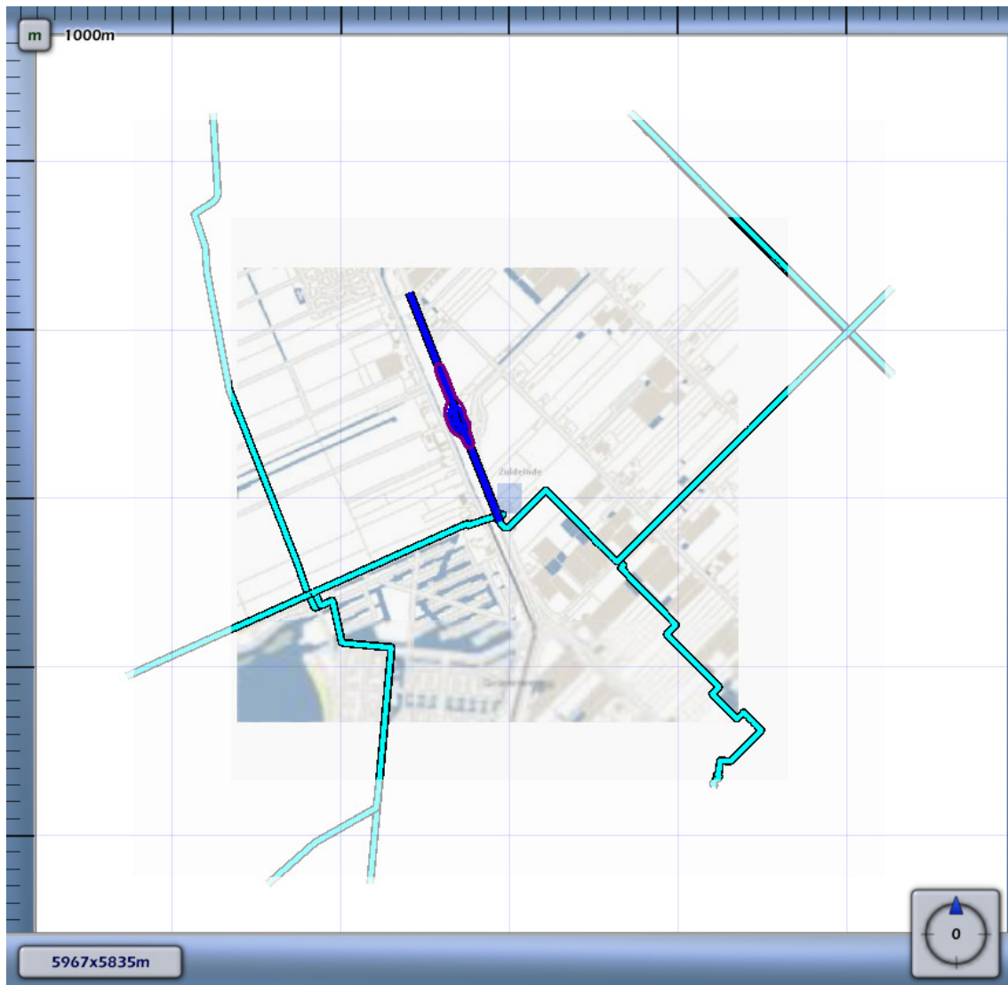
3.9 Figuur 3.9 Plaatsgebonden risico voor 398_leiding-W-521-25-deel-1 van N.V. Nederlandse Gasunie
